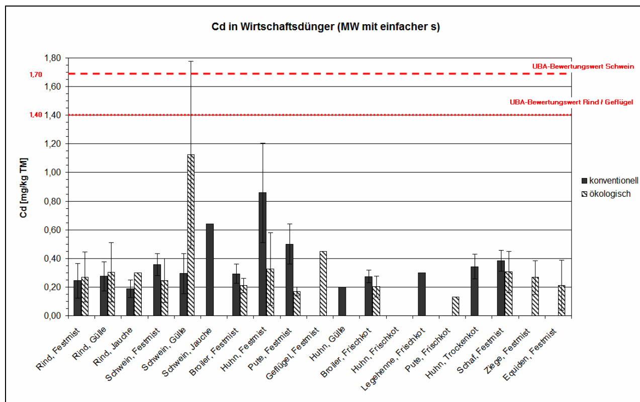
Abbildung I.5: Cd-Gehalte in konventionellen und ökologischen Wirtschaftsdüngern (aggregierte oder einfache Mittelwerte mit einfacher Standardabweichung)
