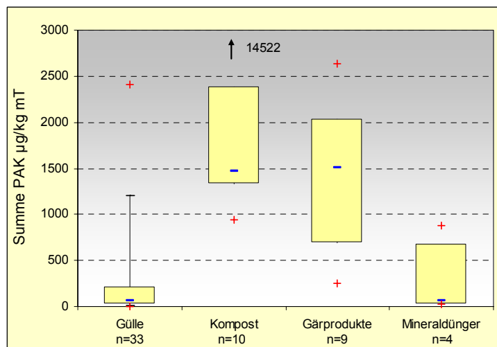
Abbildung I.29: Verteilung der PAK-Gehalte (Summe PAK nach EPA) in den untersuchten Sekundärrohstoffdüngern
