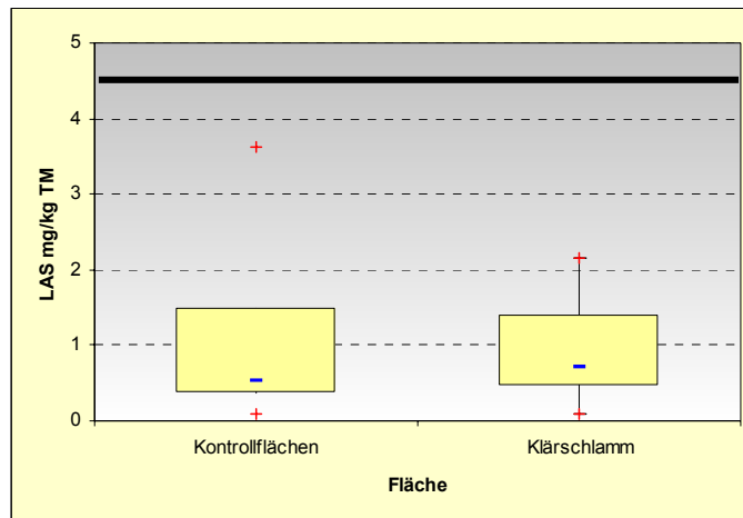
Abbildung II.5: Verteilung der LAS-Gehalte in den untersuchten Böden
