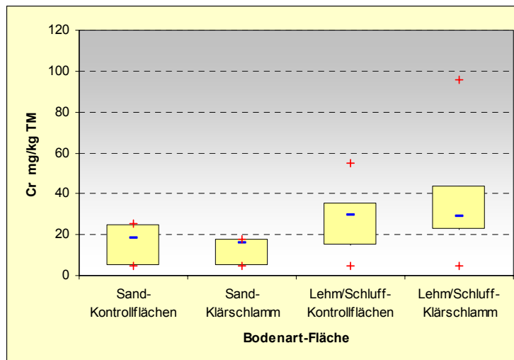
Abbildung II.10: Verteilung der Chrom-Gehalte in den untersuchten Böden
