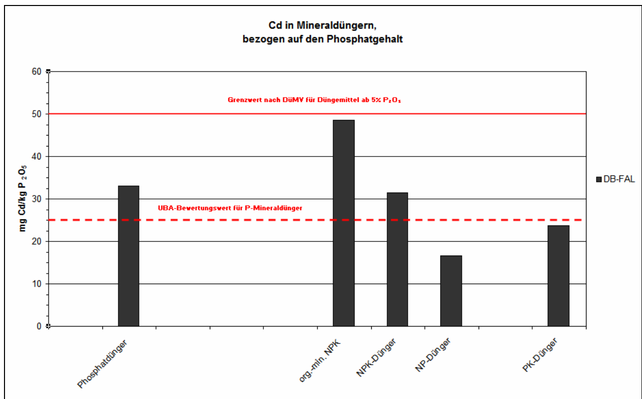
Abbildung I. 2: Mittlere Cd-Gehalte in Mineraldüngern, bezogen auf den Phosphatgehalt
