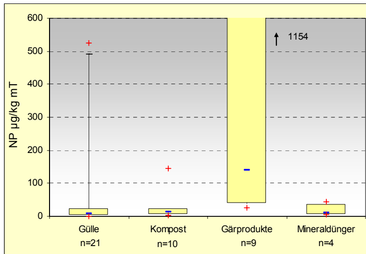
Abbildung I.24: Verteilung der 4-Nonylphenol - Gehalte in den untersuchten Sekundärrohstoffdüngern
