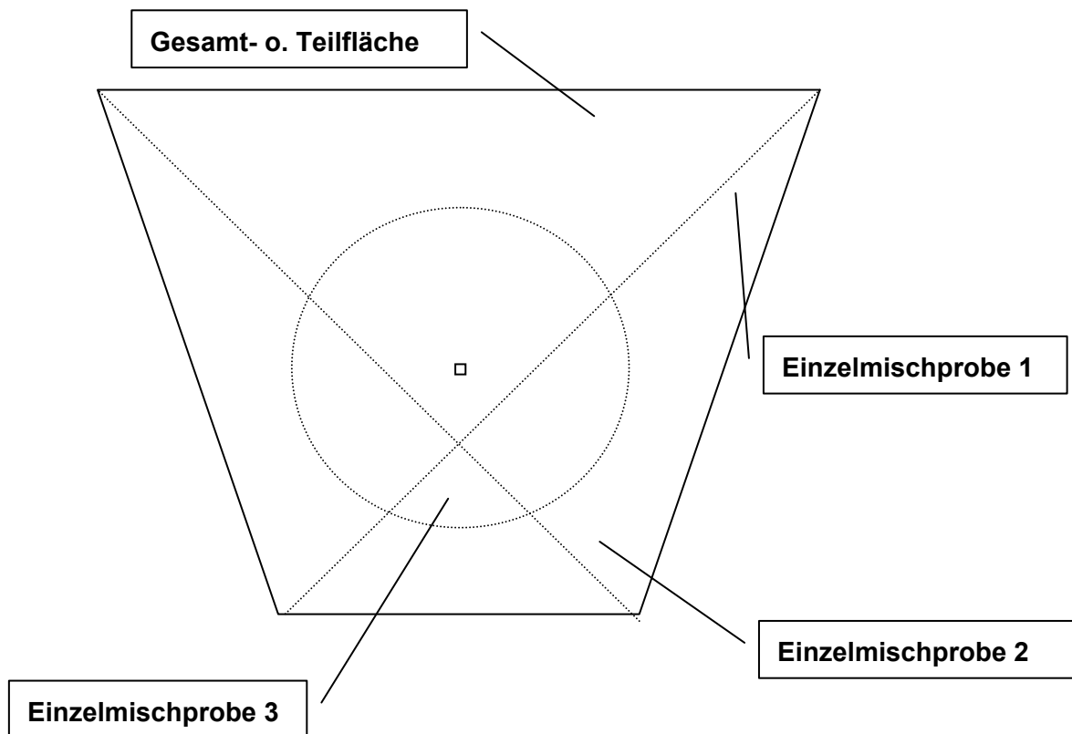
Abbildung II.3: Beprobung der Referenzflächen über Probennahmelinien
