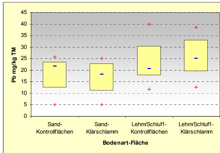
Abbildung II.9: Verteilung der Blei-Gehalte in den untersuchten Böden
