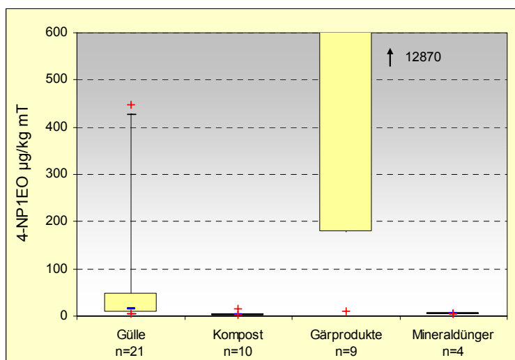
Abbildung I.25: Verteilung der 4-Nonylphenol monoethoxylat - Gehalte in den untersuchten Sekundärrohstoffdüngern
