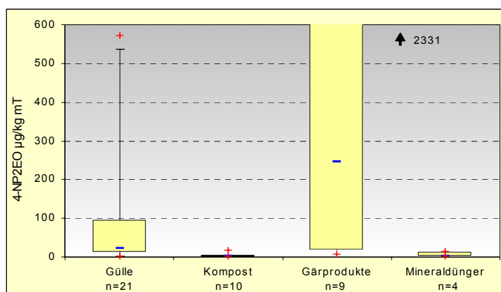
Abbildung I.26: Verteilung der 4-Nonylphenol diethoxylat - Gehalte in den untersuchten Sekundärrohstoffdüngern
