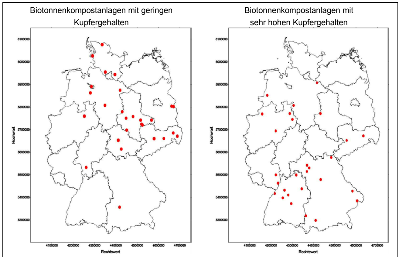
Abbildung I 30.: Standorte von Biotonnenkompostanlagen mit unterschiedlichen Kupfergehalten
