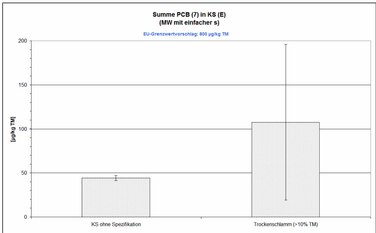
Abbildung I. 13: PCB (Summe aus 7 Kongeneren) in Klärschlamm (aggregierte oder einfache Mittelwerte mit einfacher Standardabweichung)
