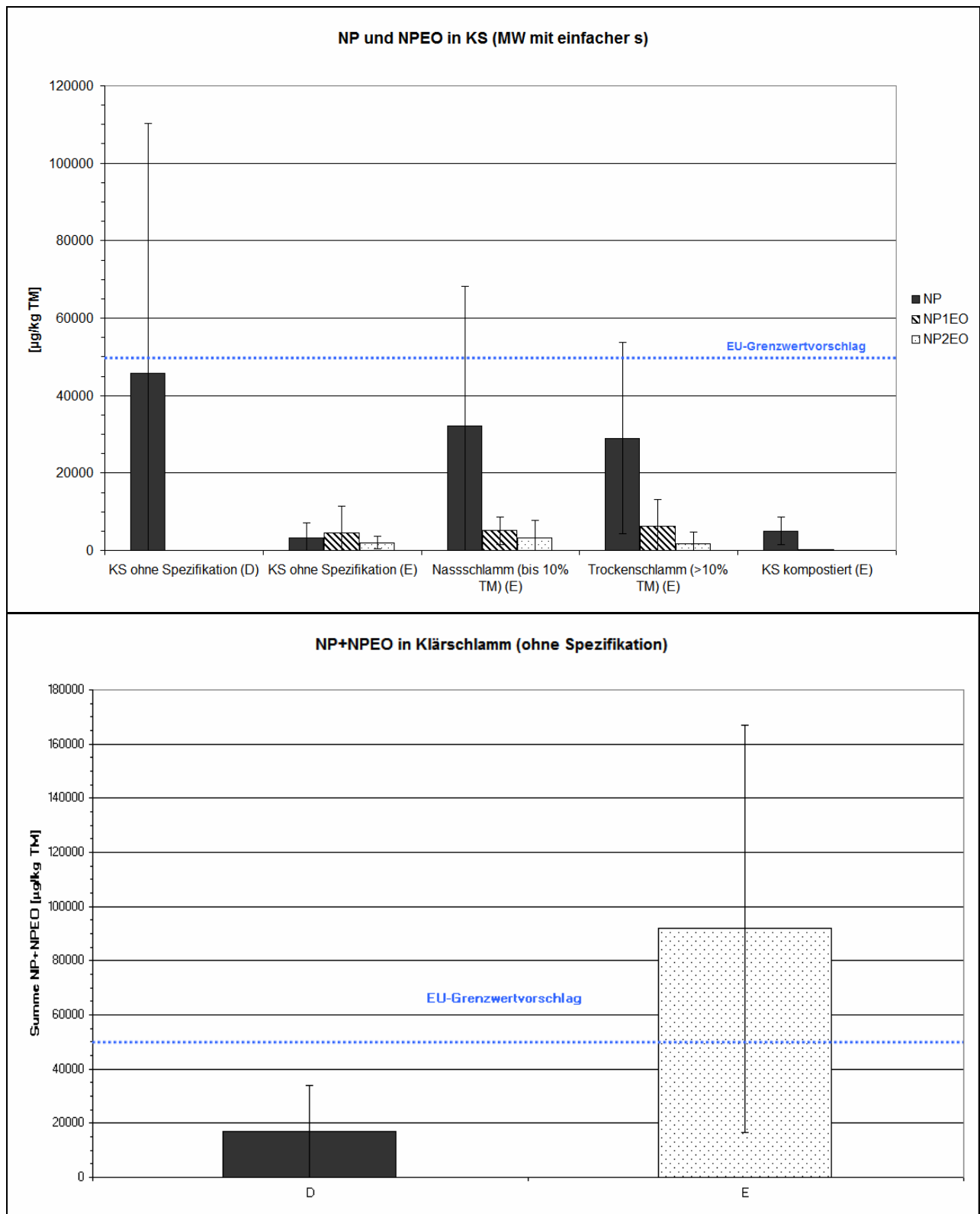
Abbildung I. 17: NP und NPEO in Klärschlamm (aggregierte oder einfache Mittelwerte mit einfacher Standardabweichung), oben: Einzelverbindungen, unten: Summe aus NP und NPEO für deutsche (D) und europäische (E) Klärschlämme
