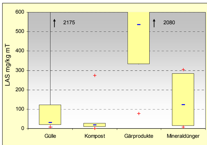
Abbildung I.23: Verteilung der LAS-Gehalte in den untersuchten Sekundärrohstoffdüngern
