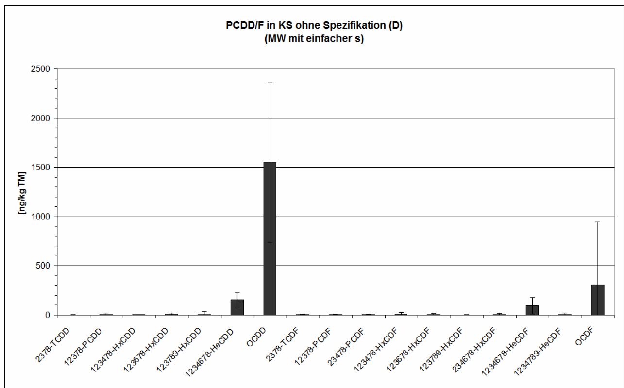
Abbildung I. 15: PCDD/F in Klärschlamm ohne Spezifikation (aggregierte oder einfache Mittelwerte mit einfacher Standardabweichung)
