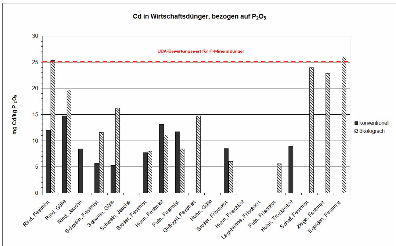
Abbildung I 6: Cd-Gehalte in konventionellen und ökologischen Wirtschaftsdüngern, bezogen auf den Phosphatgehalt
