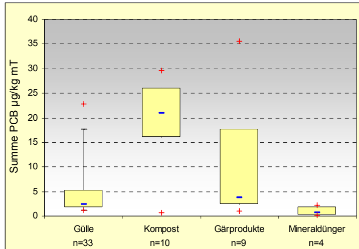
Abbildung I.28: Verteilung der PCB-Gehalte (Summe PCB) in den untersuchten Sekundärrohstoffdüngern
