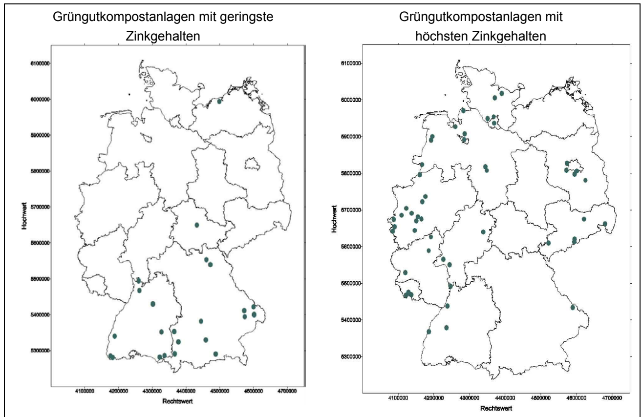
Abbildung I 31.: Anlagenstandorte von Grüngutkompostanlagen mit unterschiedlichen Zinkgehalten
