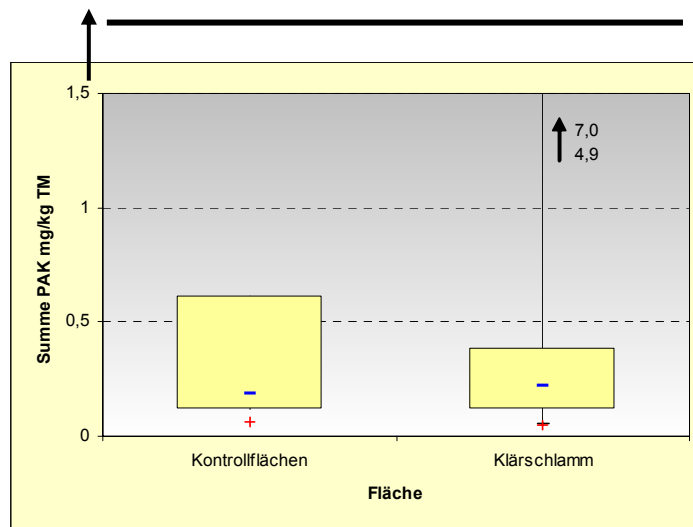
Abbildung II.4: Verteilung der PAK-Gehalte (Summe PAK nach EPA) in den untersuchten Böden
