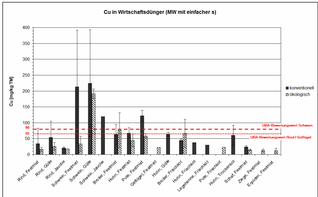
Abbildung I.7: Cu-Gehalte in konventionellen und ökologischen Wirtschaftsdüngern (aggregierte oder einfache Mittelwerte mit einfacher Standardabweichung)
