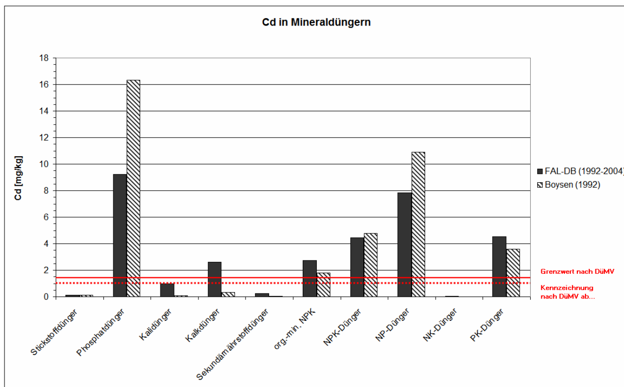
Abbildung I. 1: Cd-Gehalte in Mineraldüngern (aggregierte oder einfache Mittelwerte, mit und ohne einfache Standardabweichung) im Vergleich Boysen-Studie und FAL-Datenbank (DB)
