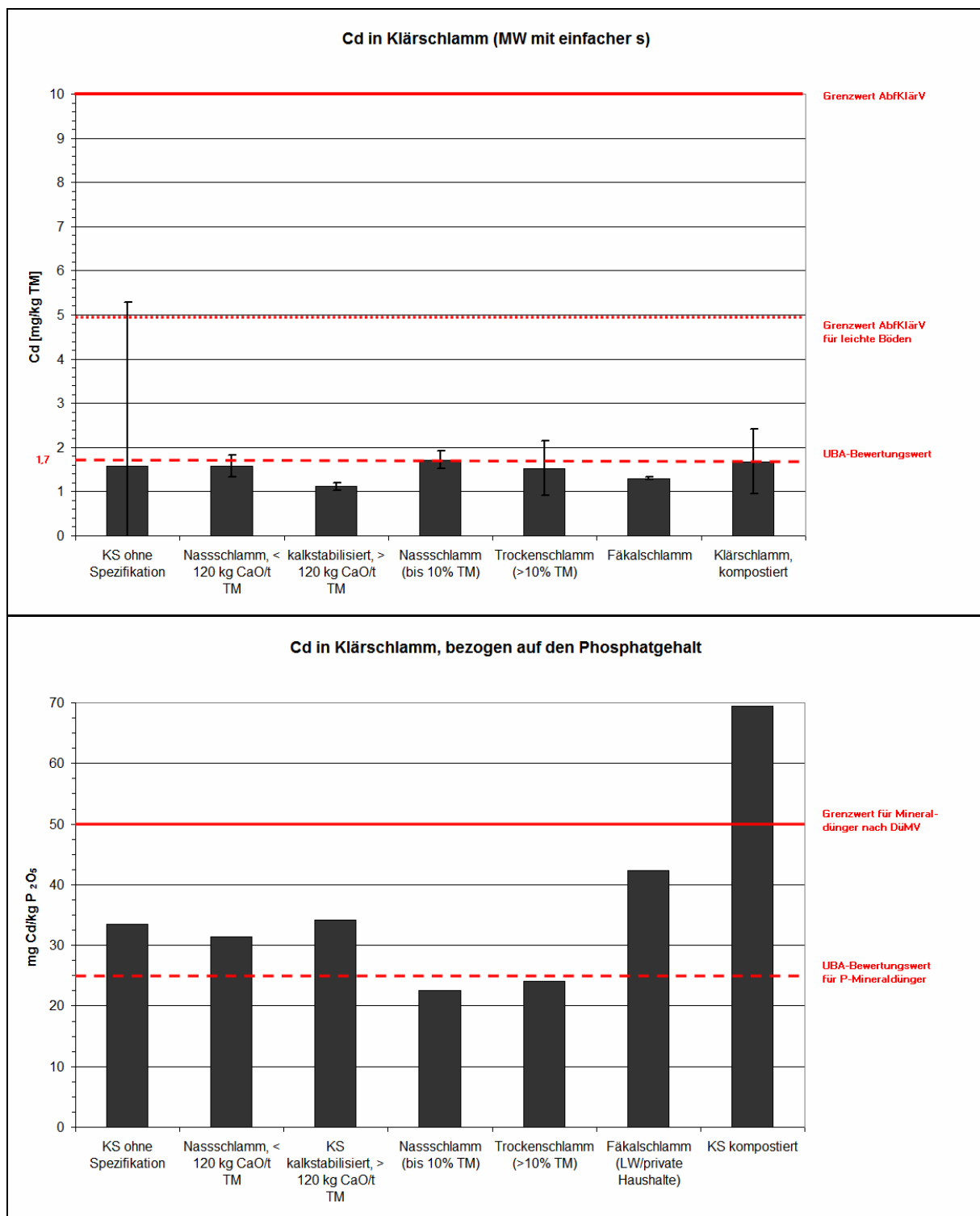
Abbildung I. 9: Cd-Gehalte in Klärschlamm, bezogen auf die Trockenmasse (aggregierte oder einfache Mittelwerte mit einfacher Standardabweichung) sowie auf den Phosphatgehalt (aggregierte Mittelwerte)
