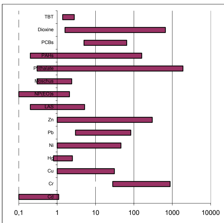
Abbildung II.2 Bereiche [mg/kg TG] für Schadstoffgehalte in landwirtschaftlich genutzten Böden nach Düngung; Ergebnisse aus der Projektphase I
