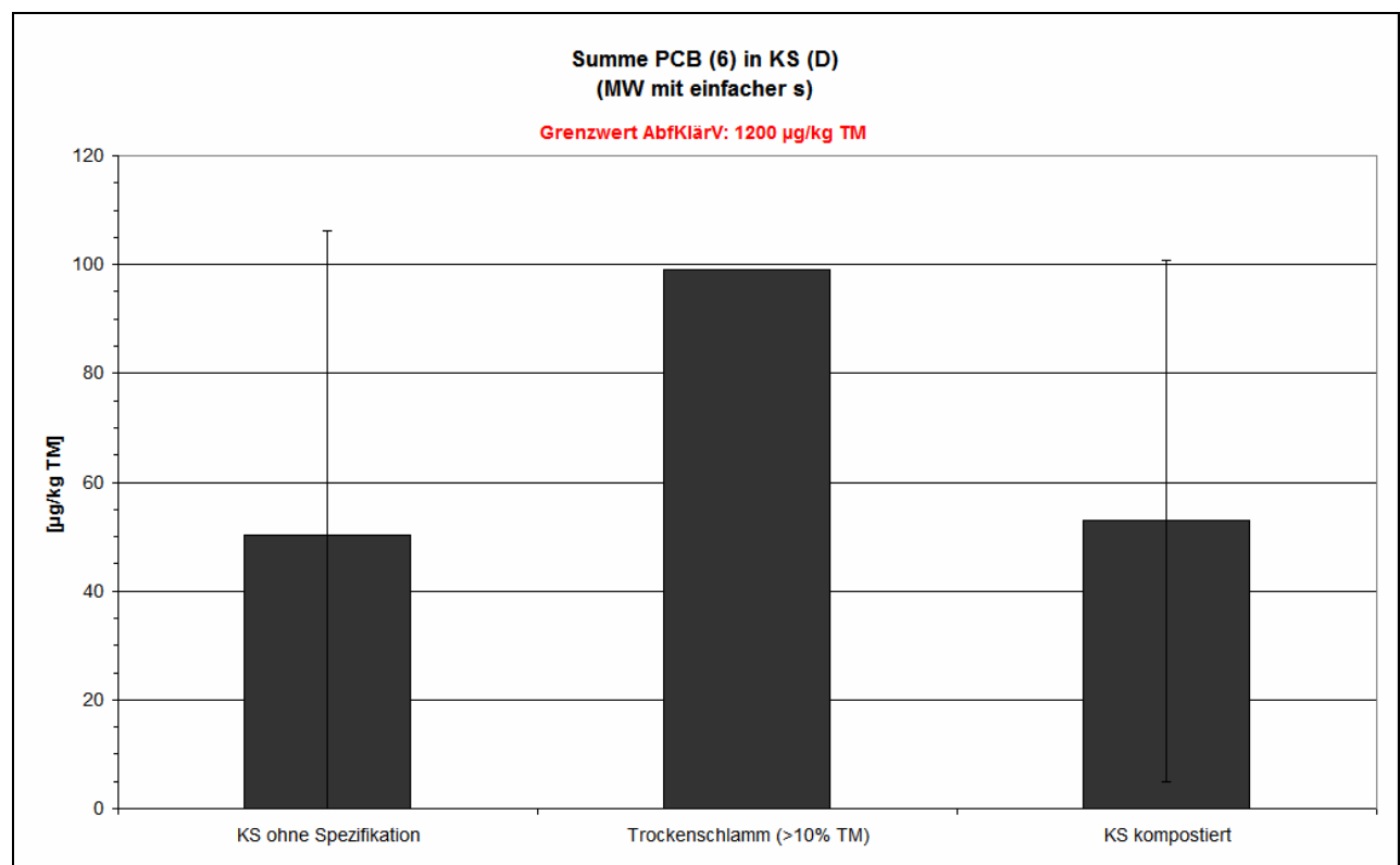
Abbildung I. 12: PCB (Summe aus 6 Kongeneren nach AbfKlärV) in Klärschlamm (aggregierte oder einfache Mittelwerte mit einfacher Standardabweichung)
