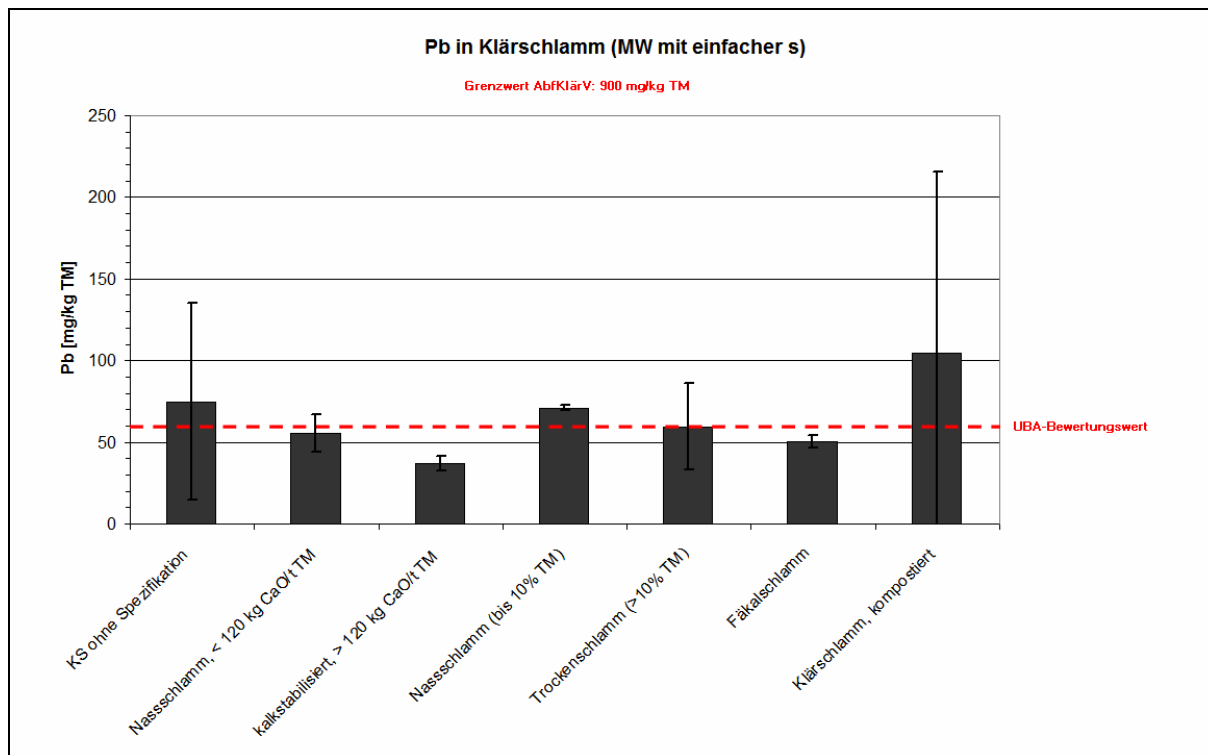
Abbildung I. 11: Pb-Gehalte in Klärschlamm (aggregierte oder einfache Mittelwerte mit einfacher Standardabweichung)
