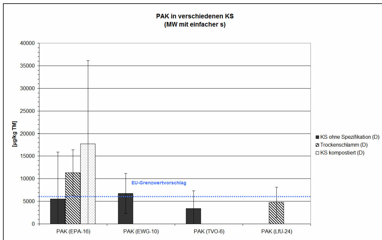
Abbildung I. 16: PAK (Summen, verschiedene Berechnungsweisen) in Klärschlamm (aggregierte oder einfache Mittelwerte mit einfacher Standardabweichung)
