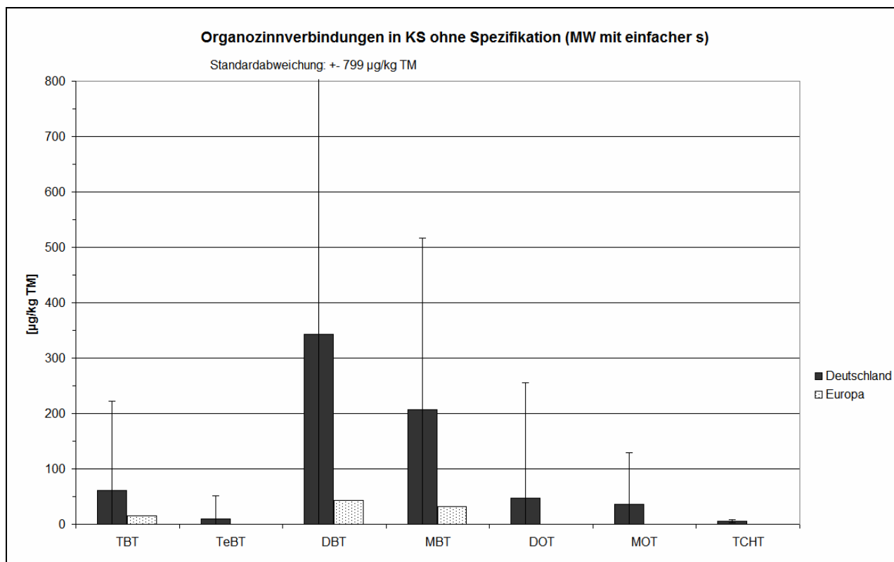
Abbildung I. 21: Organozinnverbindungen in Klärschlamm ohne Spezifikation (aggregierte oder einfache Mittelwerte mit einfacher Standardabweichung)
