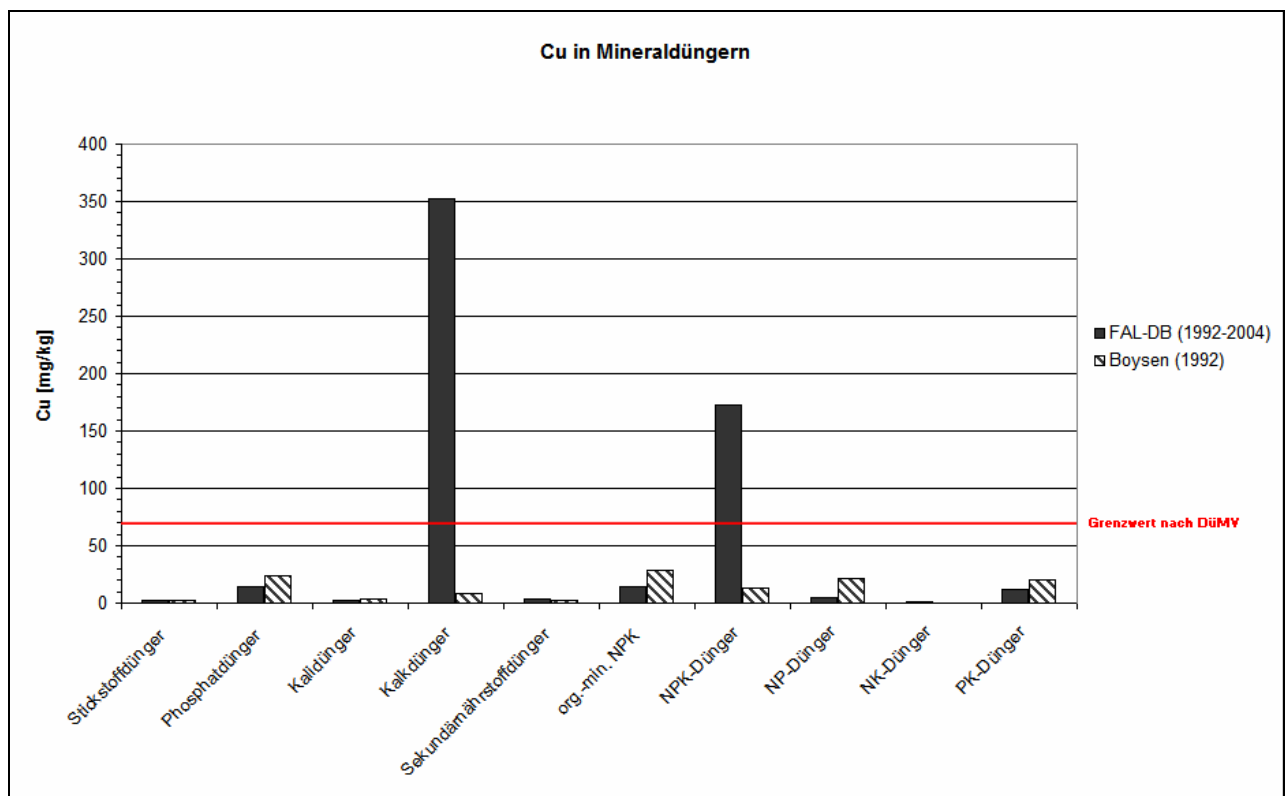
Abbildung I. 3: Cu-Gehalte in Mineraldüngern (aggregierte oder einfache Mittelwerte mit und ohne einfache Standardabweichung) im Vergleich Boysen-Studie und FAL-Datenbank (DB)
