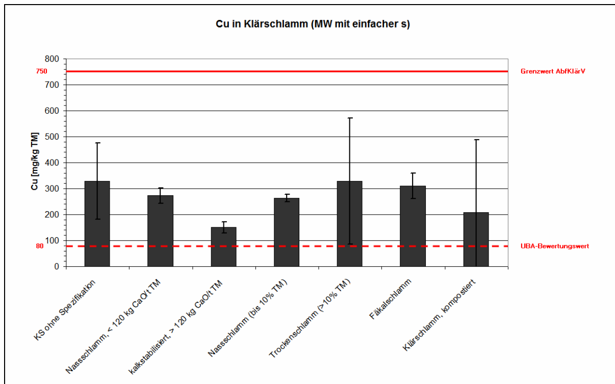
Abbildung I. 10: Cu-Gehalte in Klärschlamm (aggregierte oder einfache Mittelwerte mit einfacher Standardabweichung)
