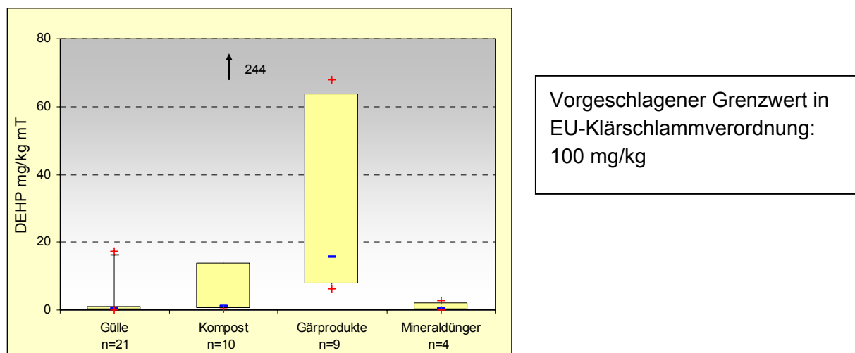
Abbildung I.27: Verteilung der DEHP-Gehalte in den untersuchten Sekundärrohstoffdüngern
