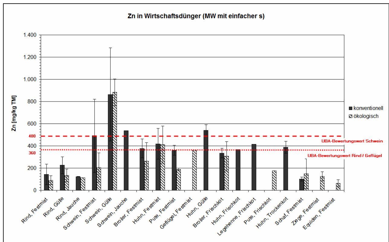
Abbildung I. 8a: Zn-Gehalte in konventionellen und ökologischen Wirtschaftsdüngern (aggregierte oder einfache Mittelwerte mit einfacher Standardabweichung)
