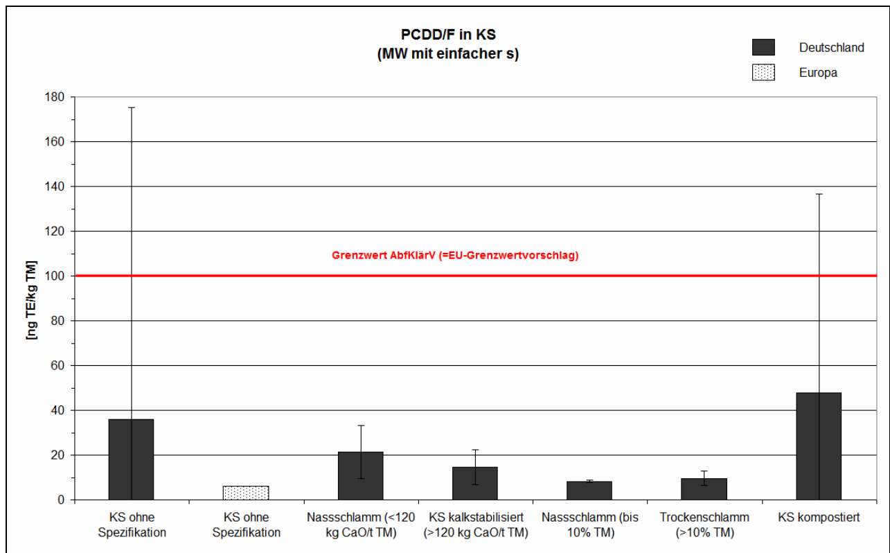
Abbildung I. 14: PCDD/F (Summe von 17 Einzelverbindungen in PCDD-Toxizitäts-Äquivalenten nach AbfKlärV) in Klärschlamm (aggregierte oder einfache Mittelwerte mit einfacher Standardabweichung)
