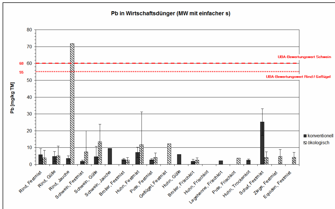
Abbildung I. 8: Pb-Gehalte in konventionellen und ökologischen Wirtschaftsdüngern (aggregierte oder einfache Mittelwerte mit einfacher Standardabweichung)
