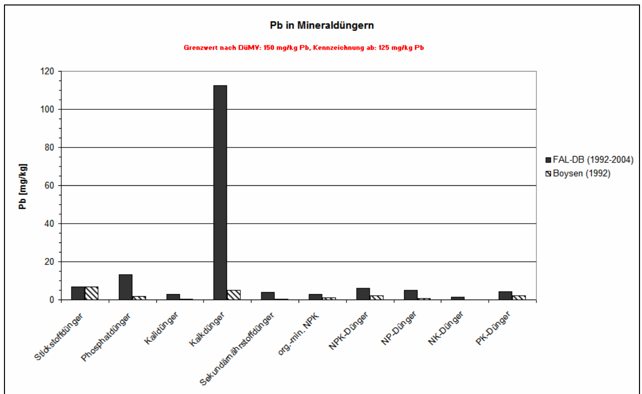
Abbildung I. 4: Pb-Gehalte in Mineraldüngern (aggregierte oder einfache Mittelwerte mit und ohne einfache Standardabweichung) im Vergleich Boysen-Studie und FAL-Datenbank (DB)
