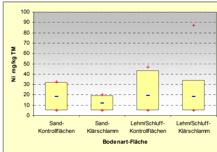
Abbildung II.12: Verteilung der Nickel-Gehalte in den untersuchten Böden
