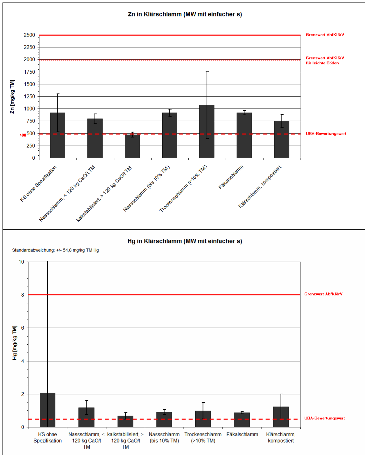
Abbildung I. 11a: Zn- und Hg-Gehalte in Klärschlamm, bezogen auf die Trockenmasse (aggregierte oder einfache Mittelwerte mit einfacher Standardabweichung)
