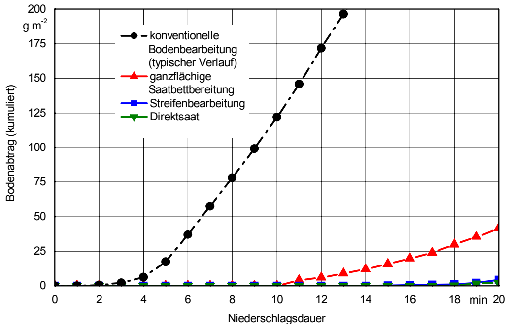
Abbildung 26: Kumulativer Bodenabtrag auf unterschiedlich bearbeiteter bzw. direkt bestellter Ackerfläche (Regensimulationsversuch, Körnermais, Lößhügelland, Beregnungsintensität: 1,9 mm/Minute)
