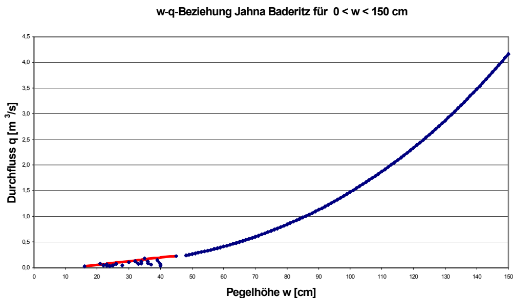
Abbildung 15: Pegelschlüsselkurve (Abflusskurve) des Pegels Jahna (Multisensormodul-Messstation)
