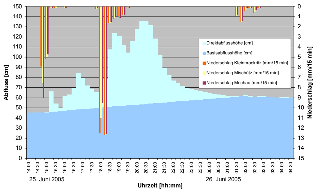
Abbildung 14: Pegel Jahna: Beobachtete Abflussganglinien für das Niederschlags-Abfluss-Ereignis am 25. Juni 2005. Die Trennung zwischen Direkt- und Basisabfluss ist geschätzt
