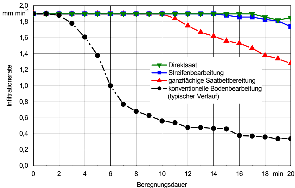
Abbildung 25: Wasserinfiltration auf unterschiedlich bearbeiteter bzw. direkt bestellter Ackerfläche (Regensimulationsversuch, Körnermais, Lößhügelland, Beregnungsintensität: 1,9 mm/Minute)
