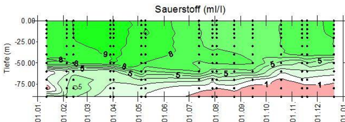
Abb. 30: Sauerstoffverhältnisse im Bornholmtief (Station 213) im Jahr 2012 - IOW- und SMHI-Daten
