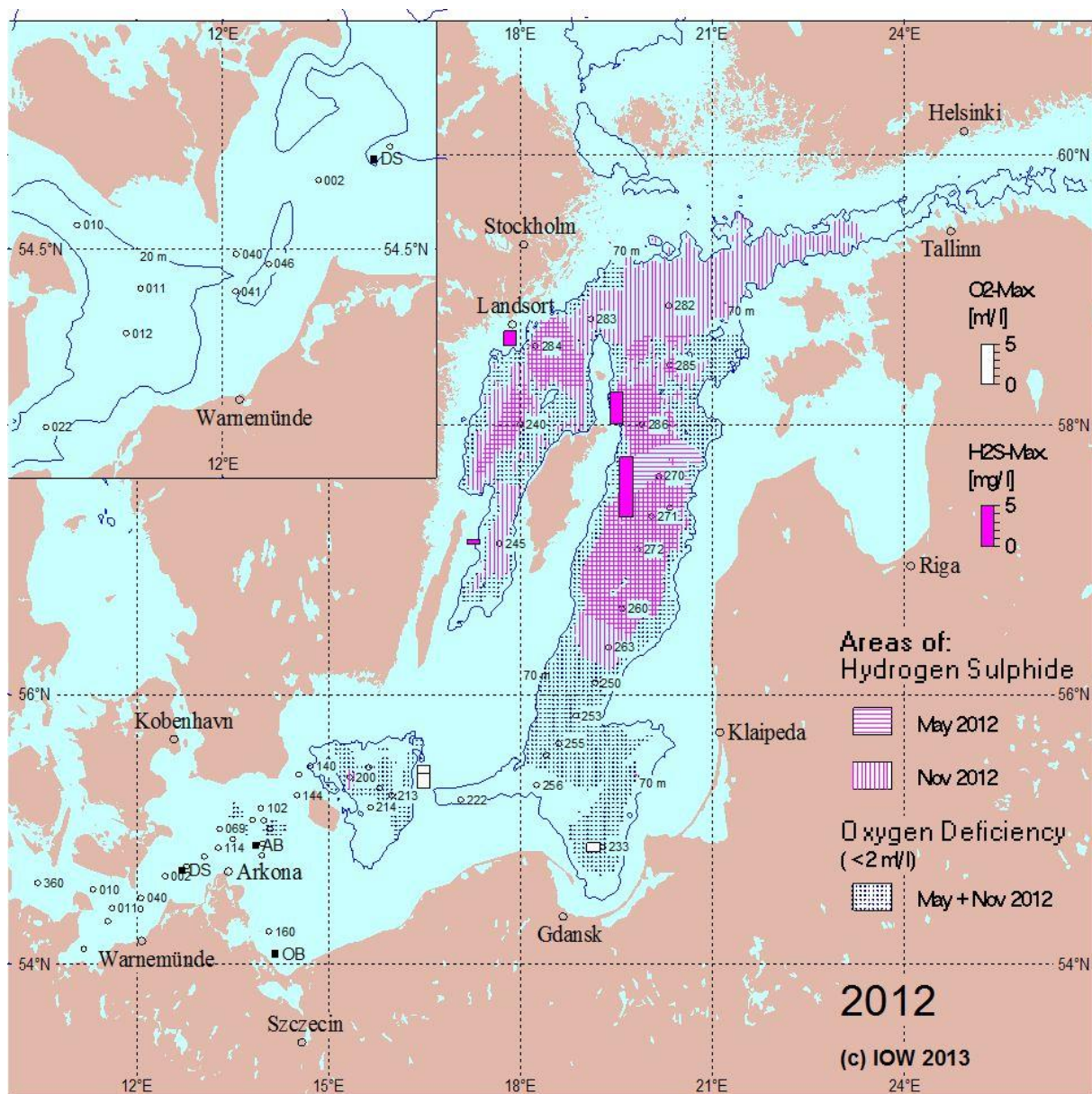
Abb. 1: Stationskarte (■ MARNET-Stationen) und Gebiete mit Sauerstoffmangel und Schwefelwasserstoff in der grundnahen Wasserschicht der Ostsee sowie maximale Sauerstoff- und Schwefelwasserstoffkonzentrationen an ausgewählten Stationen (Säulen) im Jahre 2012; die Abb. enthält zusätzlich die 70 m - Tiefenlinie bzw. die 20 m -Tiefenlinie (Bildausschnitt)
