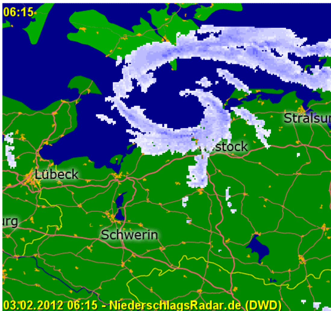
Abb. 3: Tiesel-Zyklone „Katarzyna“ über der Ostsee mit Wolkenspirale (Schneefall) während des extremen Kälteeinbruchs im Februar 2012 durch das russische Hoch „Dieter“. Niederschlagsradarbild des DWD im Internet
