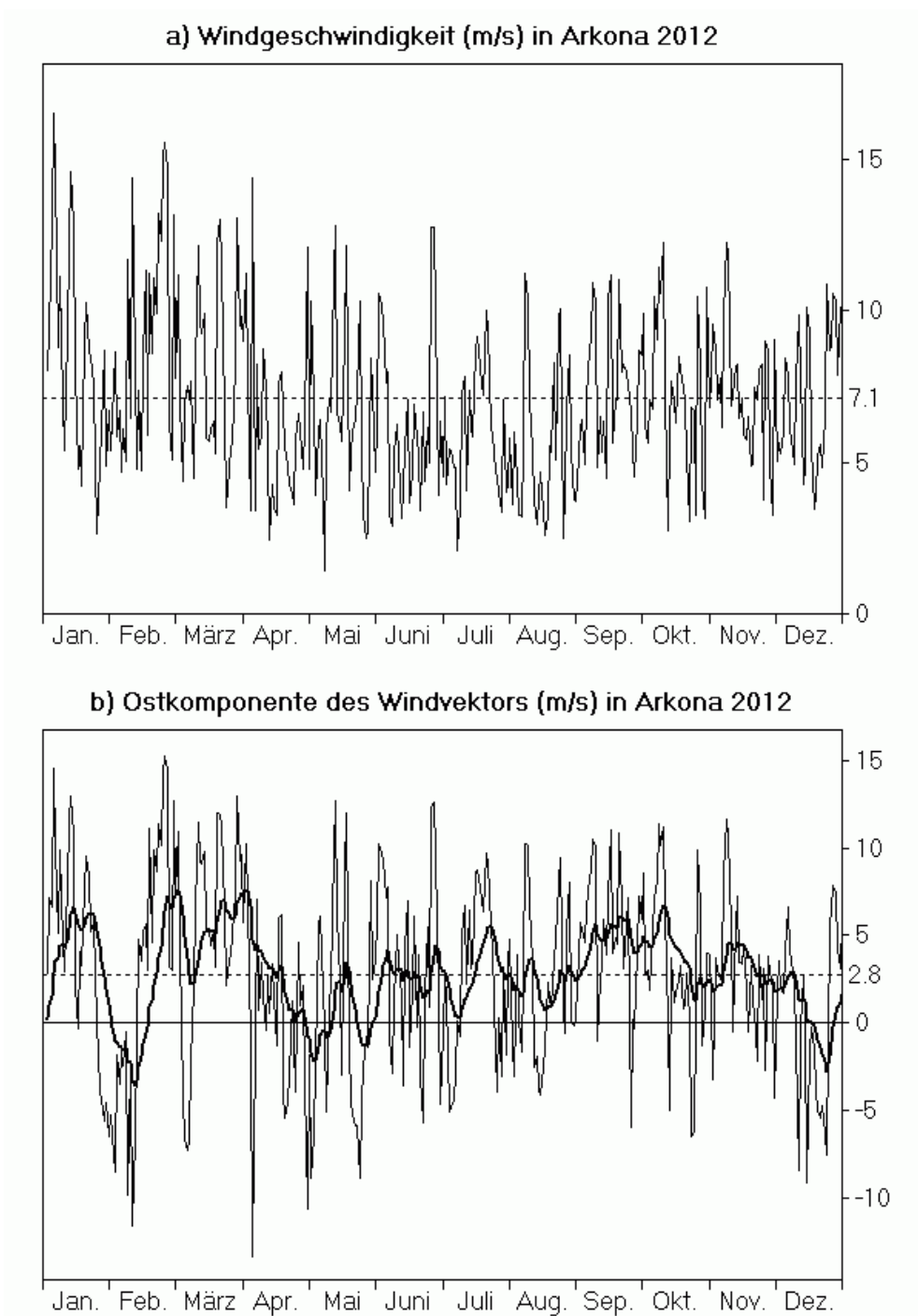
Abb. 5: Windmessungen an der Wetterstation Arkona (nach Daten des DWD, 2013b). a) Tagesmittelwerte der Windgeschwindigkeit in m/s, Jahresmittelwert 7,1 m/s gestrichelt. b) Tagesmittelwerte der Ostkomponente (Westwind positiv), Jahresmittelwert 2,8 m/s gestrichelt. Die fett gezeichnete Linie ist mit einem exponentiellen Gedächtnis von 10 Tagen gefiltert
