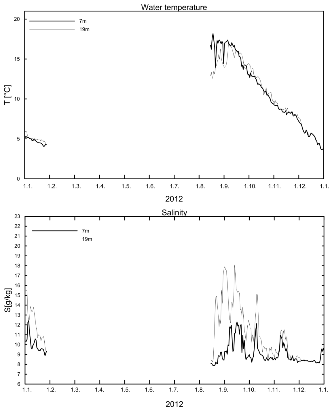
Abb. 9: Verlauf der Wassertemperatur (A) und des Salzgehaltes (B) in der Deck- und Bodenschicht auf der Darßer Schwelle im Jahre 2012
