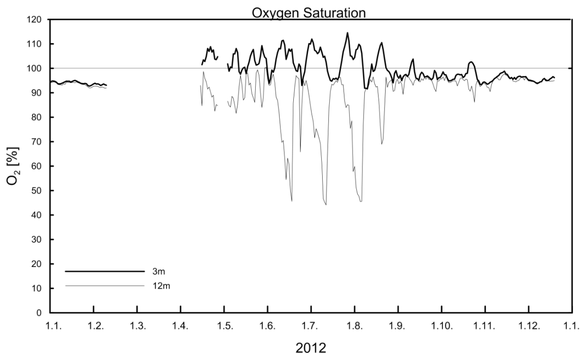
Abb. 14: Verlauf der Sauerstoffgehaltes in der Deck- und Bodenschicht in der Pommerschen Bucht (Stat. OB) im Jahr 2012
