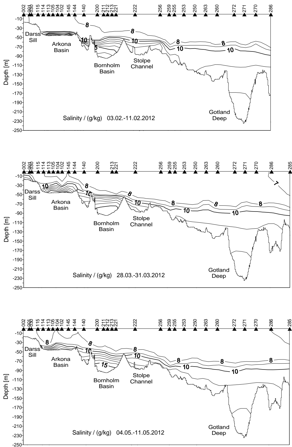
Abb. 23: Vertikale Verteilung des Salzgehaltes zwischen Darßer Schwelle und nördlichem Gotlandbecken
