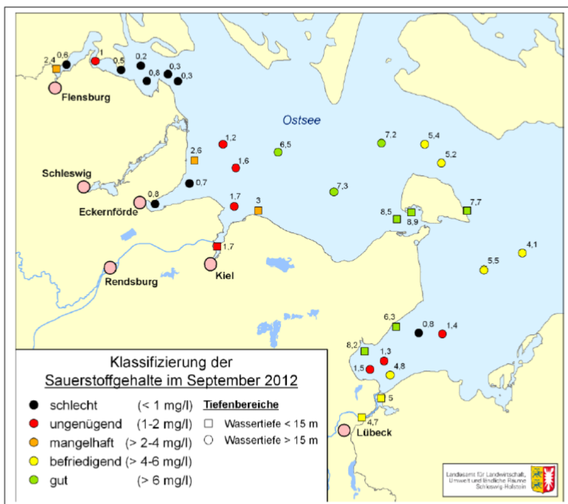
Abb. 26: Sauerstoffmangel in der westlichen Ostsee im September 2012 (LLUR, 2012) – mg/l x 0,7005 = ml/l
