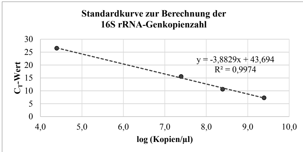
Abbildung 7: Zur Berechnung der Kopienanzahl herangezogene lineare Regression der logarithmierten Kopienanzahl/μl Template-DNA und dem mittels RT-qPCR ermittelten C T -Wert einer dekadischen Verdünnungsreihe des 16S rRNA-Gens des Referenzorganismus E. coli E2.
