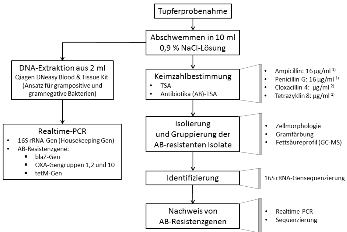
Abbildung 4: Schematischer Versuchsaufbau zur Bestimmung des Resistenzstatus in den Biofilmpuben aus der Melkanlage. Links: molekularbiologischer Ansatz, rechts: kultivierungsgestützter Ansatz.
