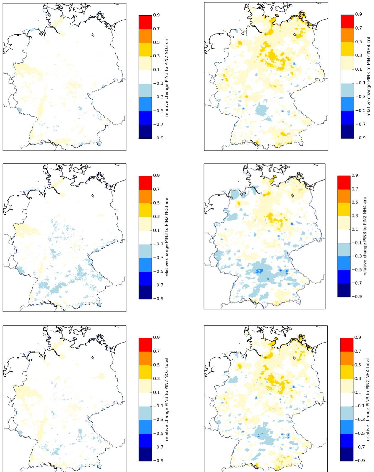
Abbildung 36. Unterschied zwischen den endgültigen Ergebnissen nach PINETI-3 und PINETI-2 für NO y (links) und NH x (rechts) bei Nadelwald (oben), Ackerland (Mitte) und der tatsächlichen Landnutzung in Deutschland (unter Einbeziehung der Messwerte der nassen Deposition)
