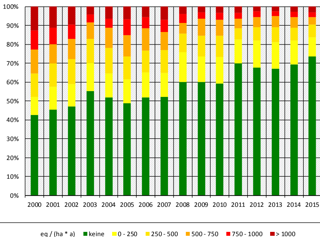
Abbildung 53: Überschreitung der Critical Load-Funktion durch Säureeinträge in den Jahren 2000 bis 2015
