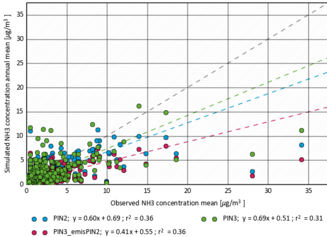
Abbildung 38: Vergleich der LOTOS-EUROS-Ergebnisse im PINETI-3-Verfahren mit den Luftkonzentrationsmesswerten für \text{NH}_3 .
