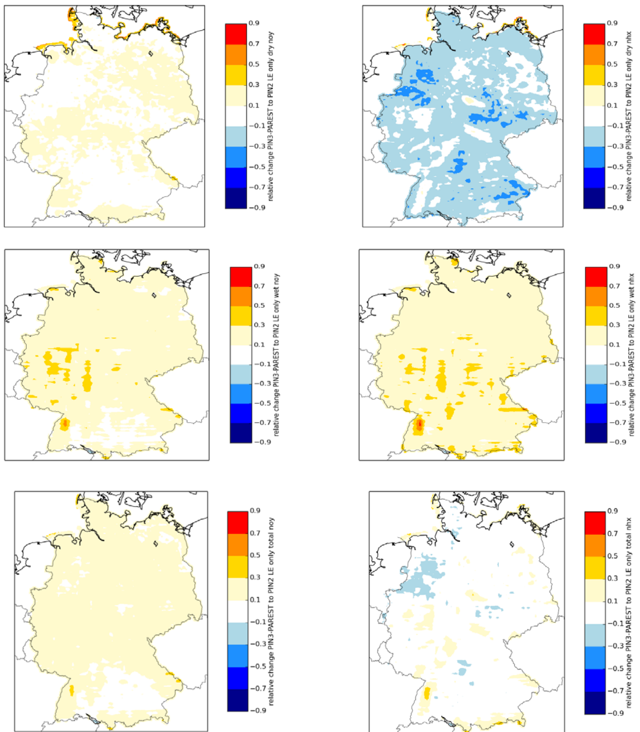
Abbildung 29. Relative Veränderung der trockenen (oben), nassen (Mitte) und Gesamtd deposition (unten) für NO y (links) und NH x (rechts) im LOTOS-EUROS-Modell v2.1 von PINETI-3 und LOTOS-EUROS v1.1.10 in PINETI-2 am Beispiel des Jahres 2009
