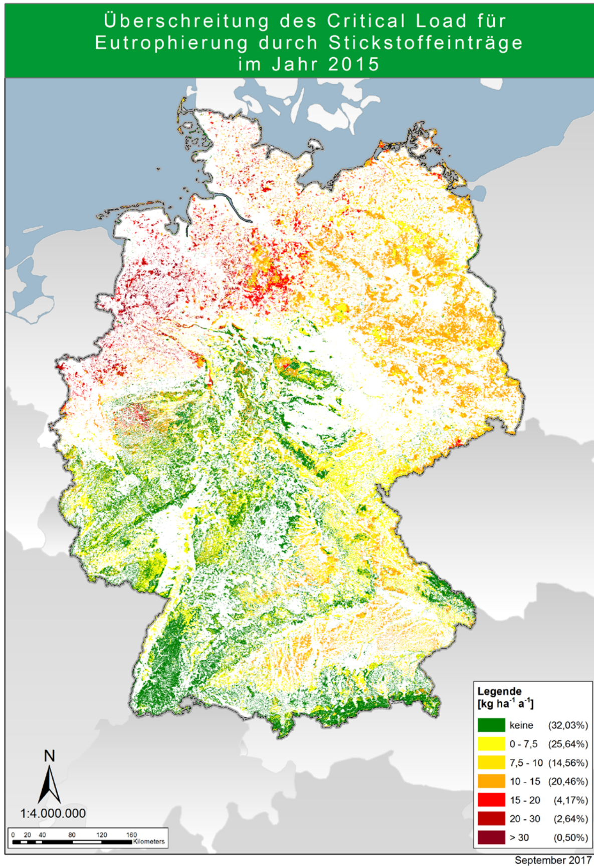
Abbildung 54: Überschreitung der Critical Load für eutrophierenden Stickstoff im Jahr 2015
