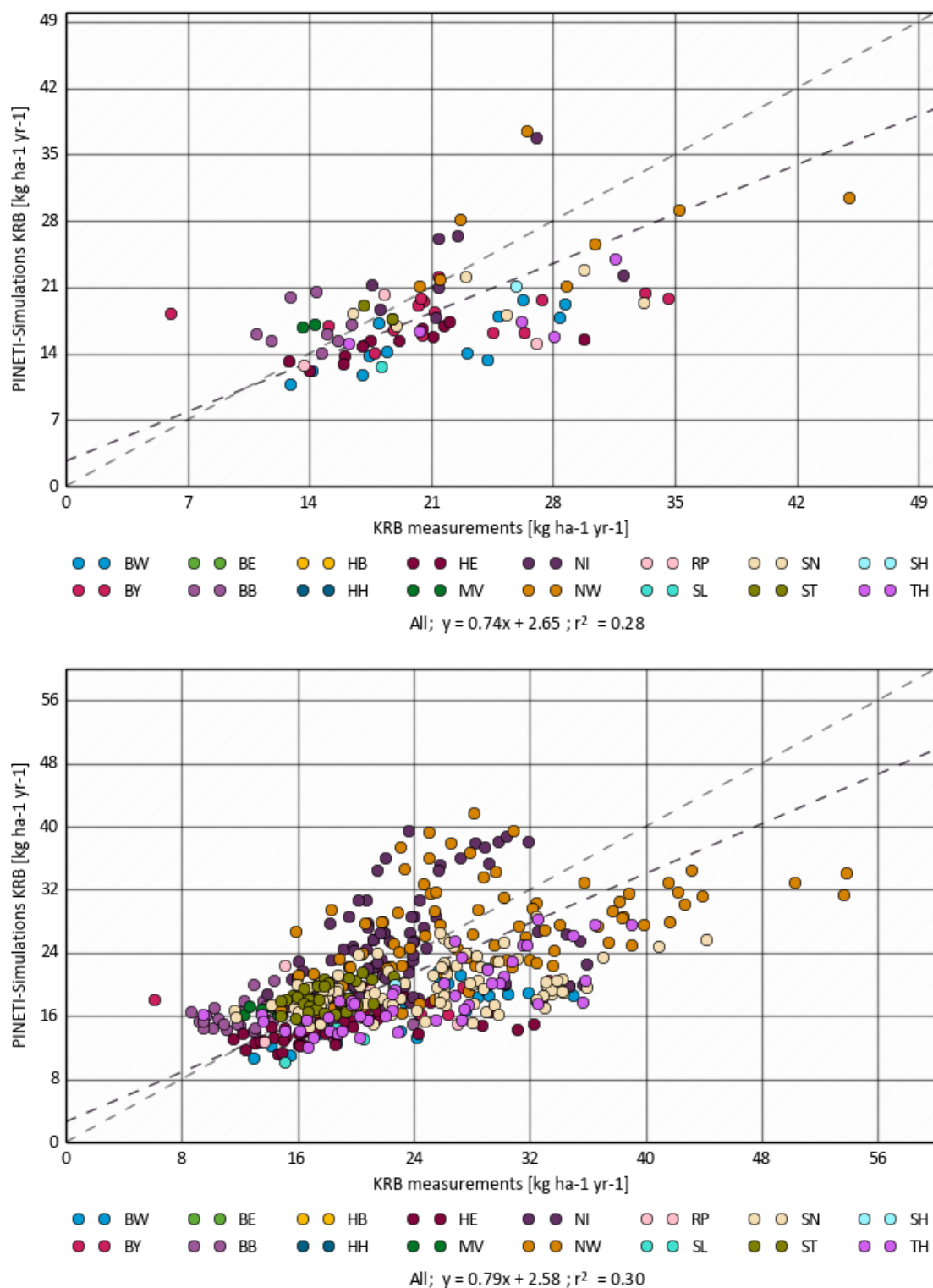
Abbildung 43: Vergleich der KRB-Ergebnisse (Methode de Vries, 2001) mit den PINETI-3-Ergebnissen. Oben: Durchschnittswert über den Zeitraum 2000 bis 2015 für die einzelnen Stationen; Unten: Ein Datenpunkt pro Station und Jahr
