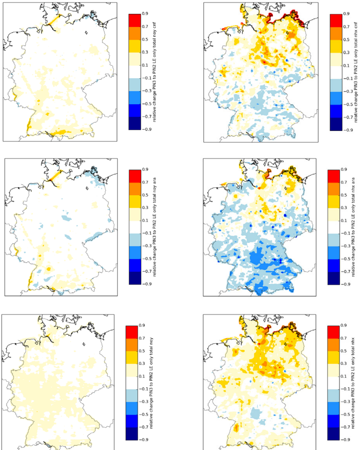
Abbildung 35. Unterschied zwischen den Ergebnissen der PINETI-3- und der PINETI-2-Modellrechnung (ohne Einbeziehung der Messwerte der nassen Deposition) für NO y (links) und NH x (rechts) bei Nadelwald (oben), Ackerland (Mitte) und der tatsächlichen Landnutzung in Deutschland
