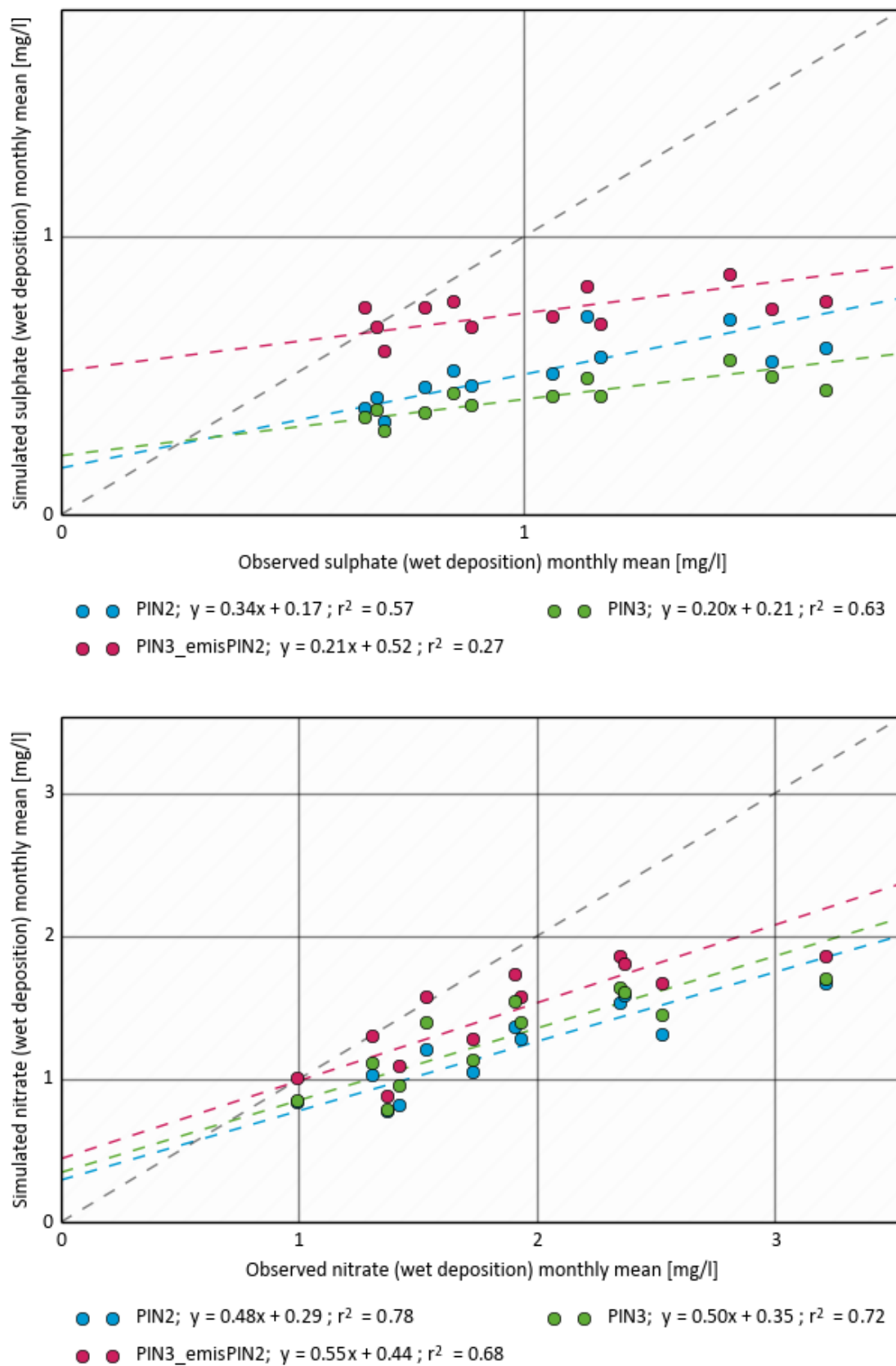
Abbildung 41: Vergleich der EMEP-Messungen für die nasse Deposition von Sulfat, Nitrat und Ammonium mit den Ergebnissen der LOTOS-EUROS-Modellrechnung
