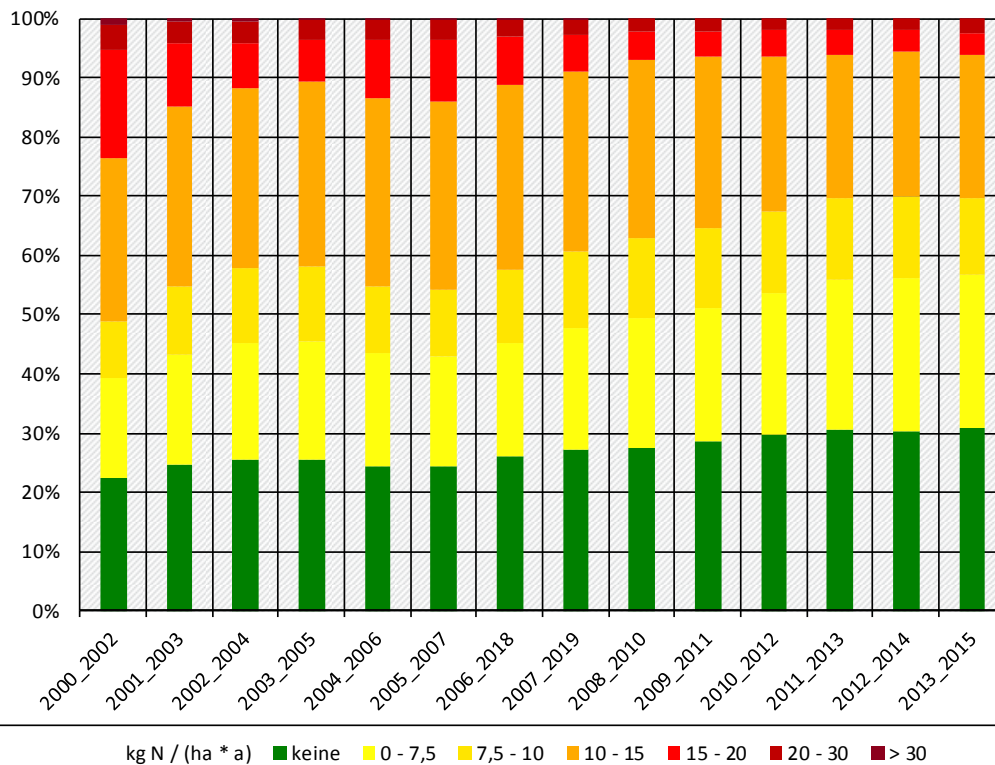
Abbildung 61: Überschreitung der Critical Load für Eutrophierung in den Jahren 2000 bis 2015 mit über drei Jahre gemittelten Eintragsraten von Stickstoff
