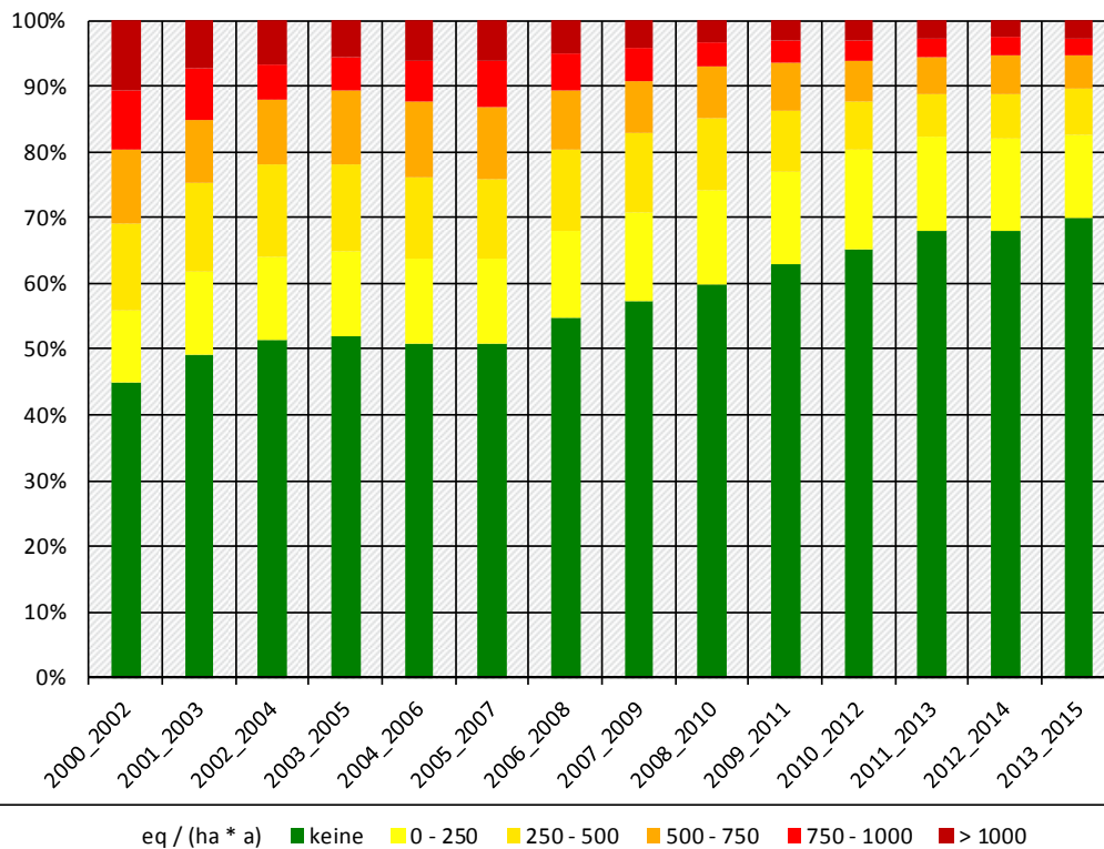
Abbildung 59: Überschreitung der Critical Load für Versauerung in den Jahren 2000 bis 2015 mit über drei Jahre gemittelten Eintragsraten von Schwefel- und Stickstoffverbindungen
