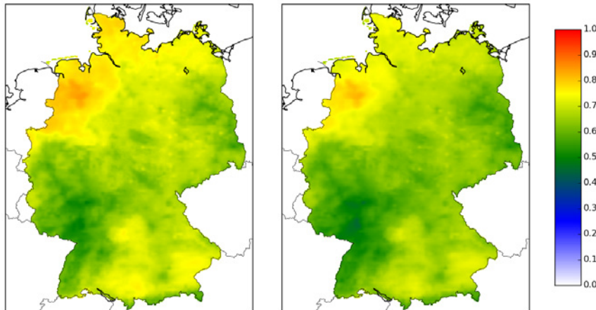
Abbildung 27. Verhältnis von \text{NH}_x zur Gesamtd deposition bei Nadelwald (links) und Gras (rechts)
