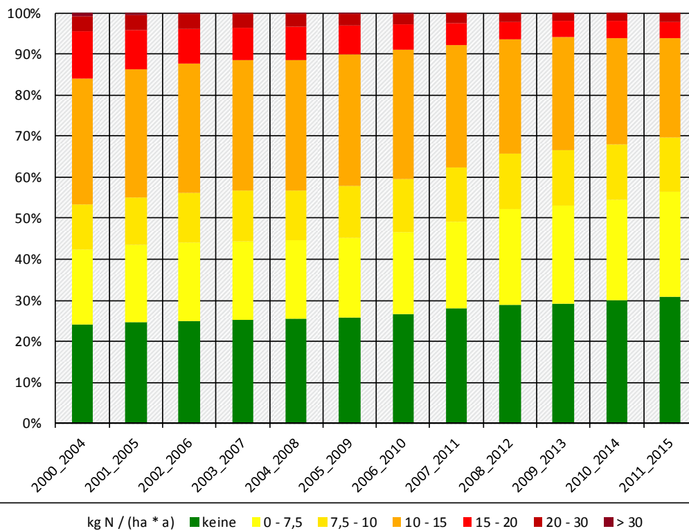
Abbildung 62: Überschreitung der Critical Load für Eutrophierung in den Jahren 2000 bis 2015 mit über fünf Jahre gemittelten Eintragsraten von Stickstoff
