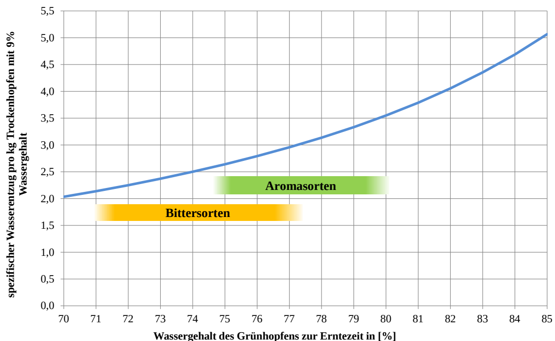
Abb. 41: Zusammenhang Wassergehalt des Grünhopfens zur Erntezeit und spezifischer Wasserentzug pro kg Trockenhopfen
