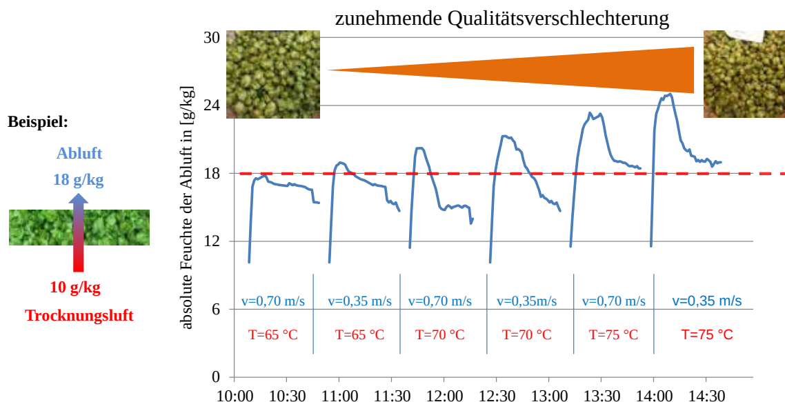
Abb. 31: Absolute Feuchte in [ \text{g}_{\text{Wasser}}/\text{kg}_{\text{Trocknungsabluft}} ] in den ersten 40min Trocknungszeit bei unterschiedlichen Trocknungstemperaturen und Luftgeschwindigkeiten
