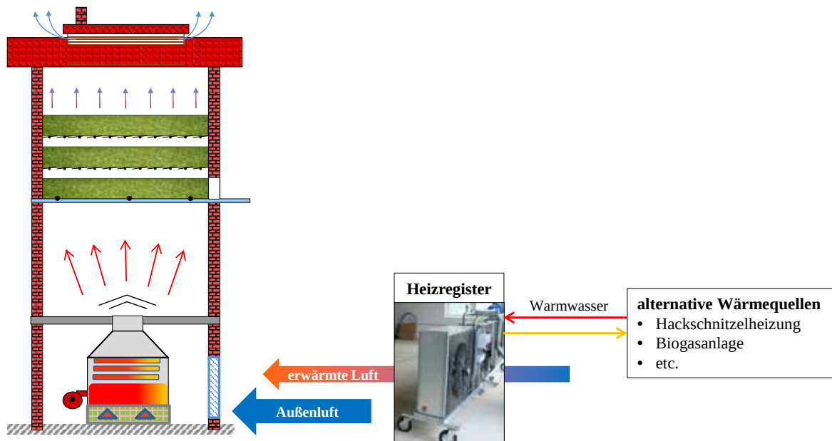
Abb. 72: Prinzip der Vorwärmung der Ansaugluft mittels Warmwasser-Heizregisters
