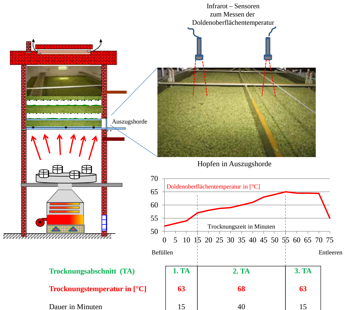
Abb. 55: Schematische Darstellung des Zusammenhangs zwischen der Temperatur der Trocknungsluft und der Doldenoberfläche des Hopfens in der Auszugshorde
