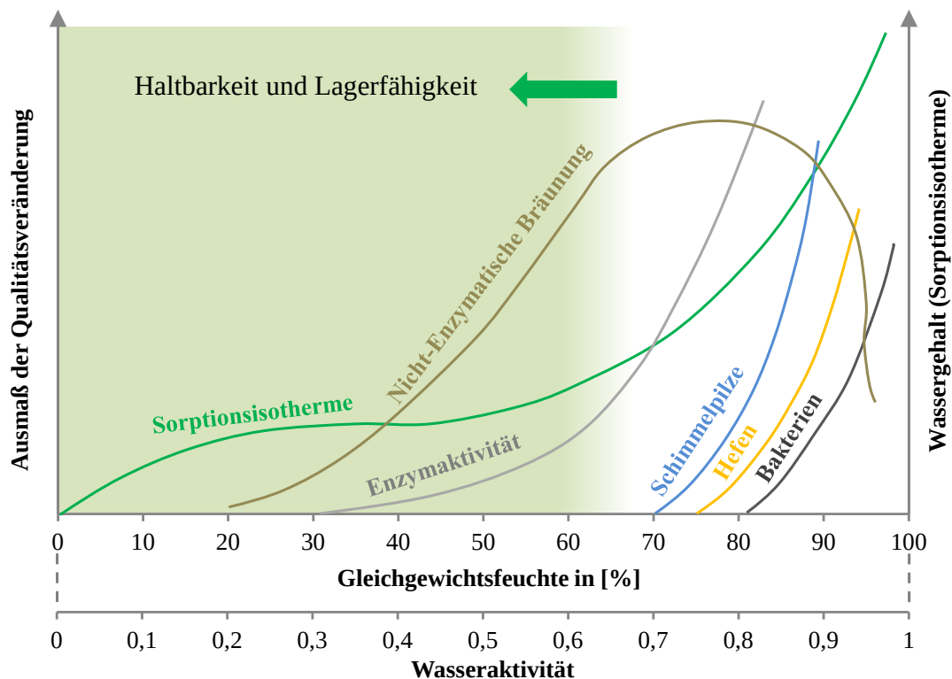
Abb. 25: Schematische Darstellung des Verlaufs der verschiedenen Verderbs-Möglichkeiten in Abhängigkeit der Gleichgewichtsfeuchtigkeit bzw. Wasseraktivität (Heiss, R. u. Eichner, K. 1971)
