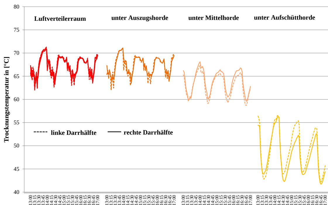
Abb. 10: Trocknungstemperaturen beim Einströmen in die unterschiedlichen Trocknungslagen auf Basis einer gleichmäßigen Wärme- und Luftverteilung
