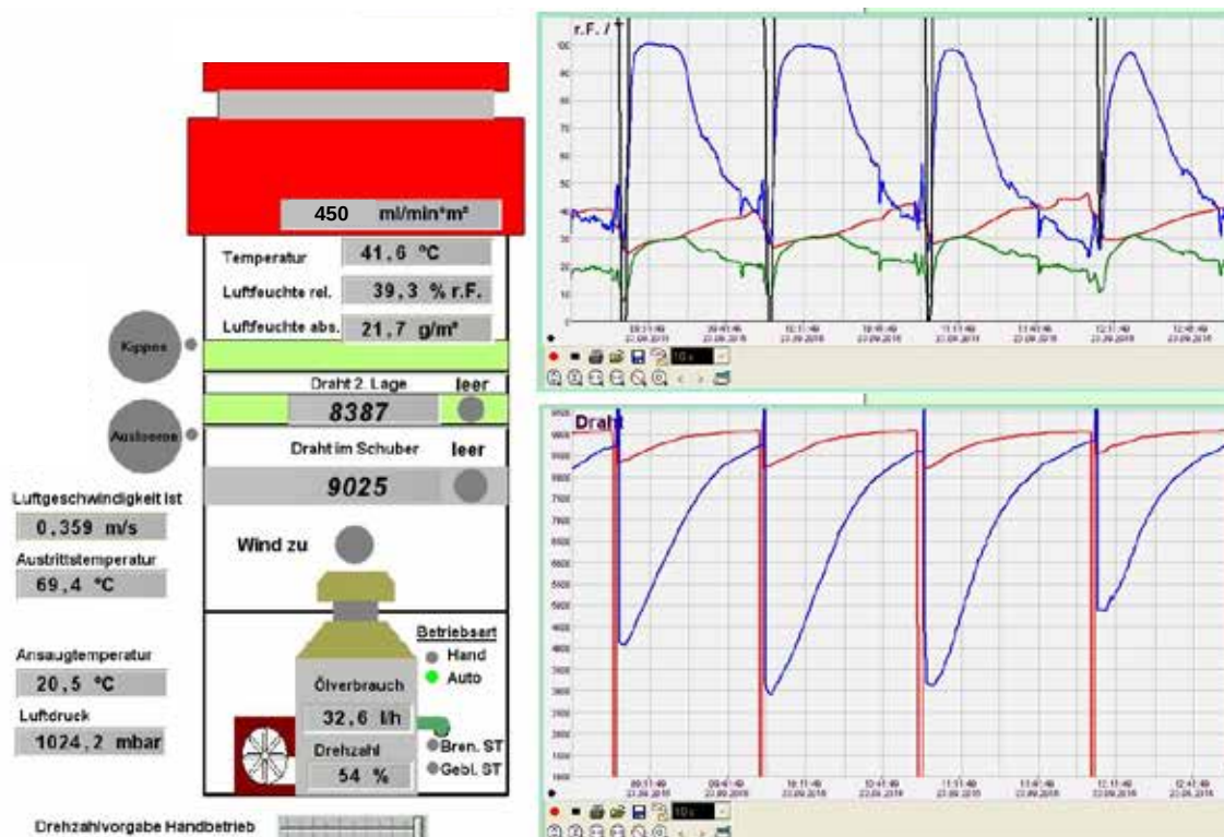
Abb. 57: Beispiel für die Anzeige und graphische Aufbereitung wichtiger Messwerte in einem Praxisbetrieb (Bild Hofer H., 2019)
