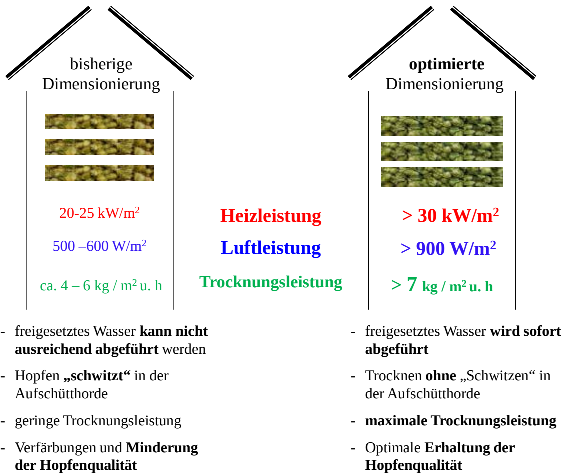
Abb. 49: Zusammenhang von Dimensionierung, Trocknungsleistung und Hopfenqualität
