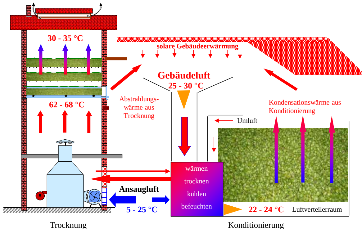
Abb. 74: Beispiel für Nutzung alternativer Energiequellen in einem Hopfenerntezentrum
