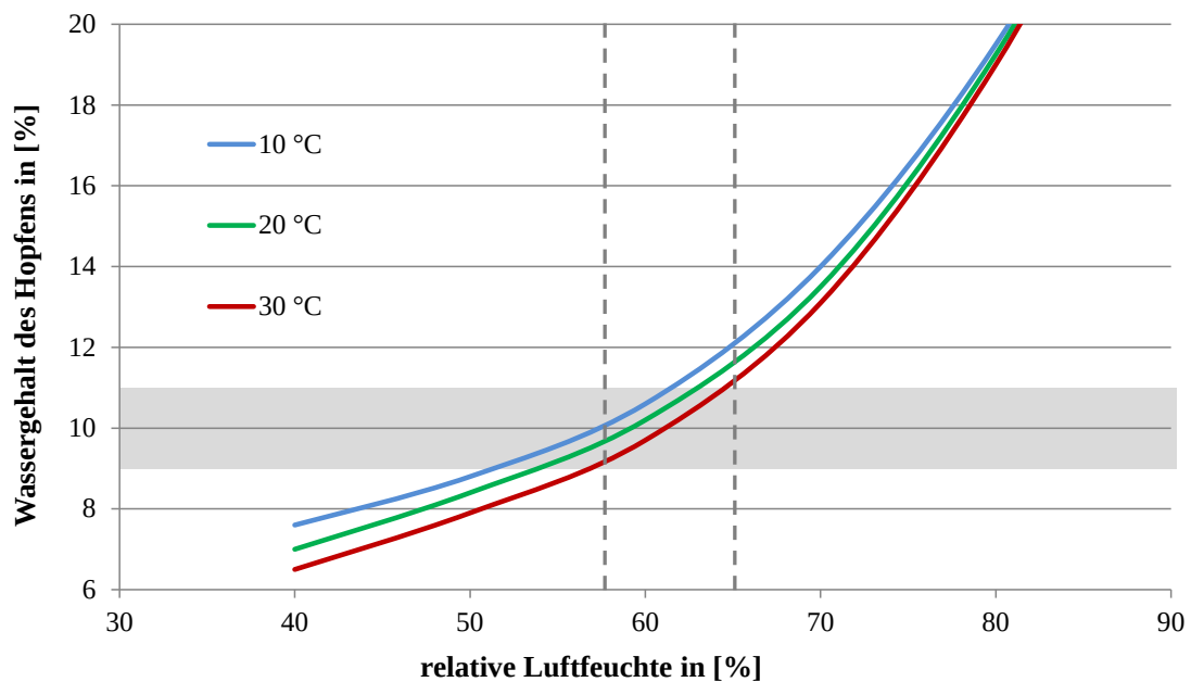
Abb. 78: Sorptionsverhalten von Hopfen
