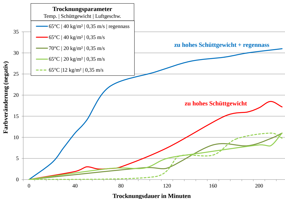
Abb. 33: Farbveränderungen bei unterschiedlichen Trocknungsbedingungen (Quelle: Dr. Barbara Sturm, Uni Kassel, 2016)
