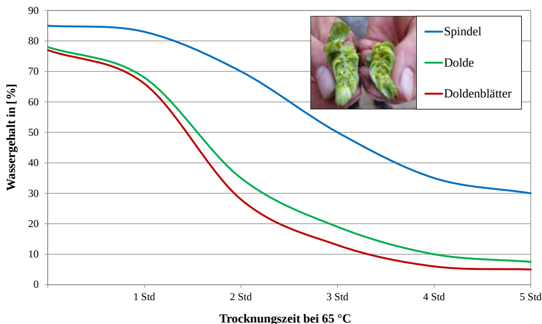
Abb. 37: Wassergehaltsabnahme während der Trocknung von Dolde, Spindel und Doldenblättern in einer Kleintrocknungsanlage
