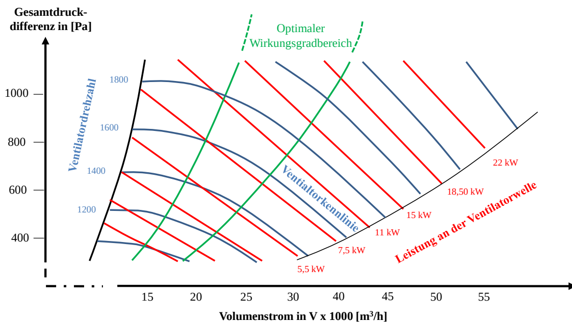
Abb. 3: Beispiel für die Ventilatorkennlinien eines Gebläses
