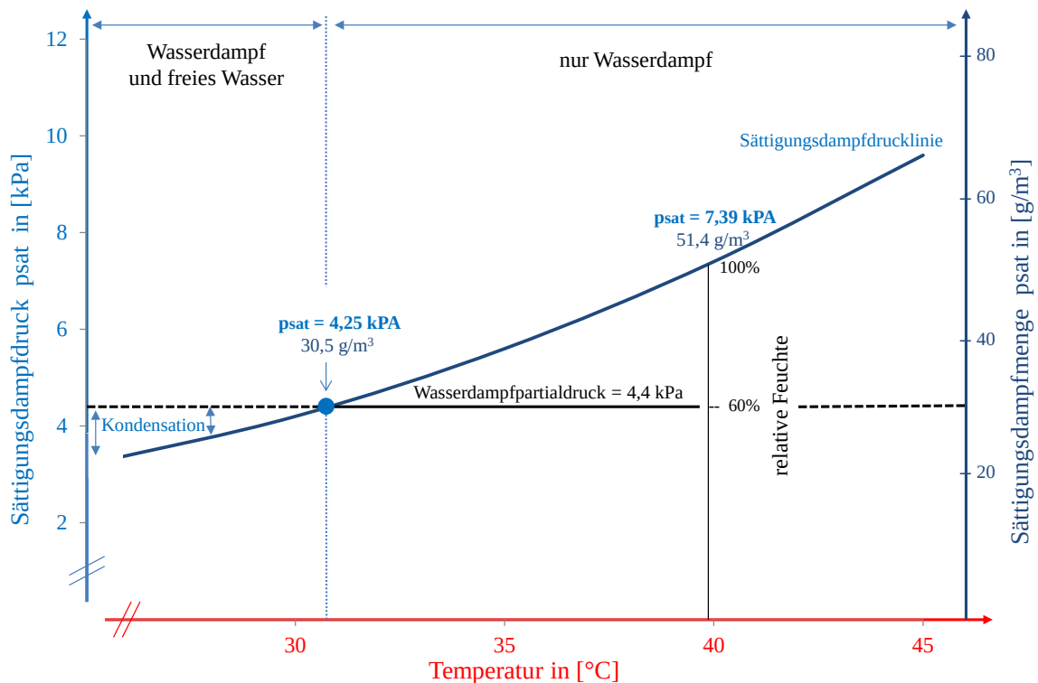
Abb. 20: Zusammenhang Sättigungsdampfdruck, Partialdruck der Luft und Kondensation
