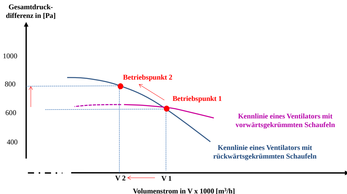
Abb. 4: Vergleich der Ventilator-kennlinien unterschiedlicher Gebläsetypen
