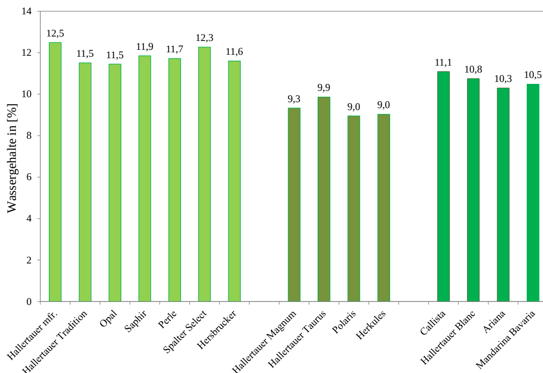
Abb. 24: Unterschiedliches Sorptionsverhalten der Hopfensorten bei gleichen Lagerbedingungen
