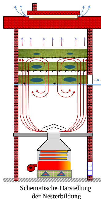
Abb. 29: Strömungsverlauf der Trocknungsluft bei Nesterbildung
