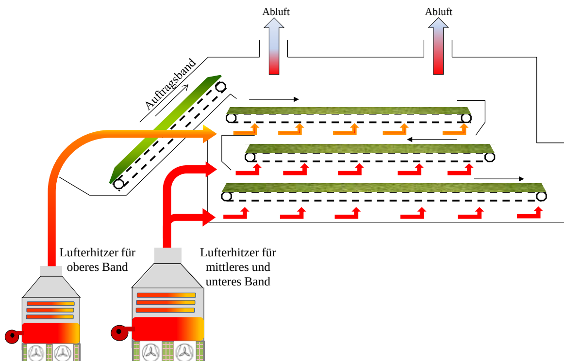
Abb. 2: Schema eines Bandtrockners mit zwei Lufterhitzern
