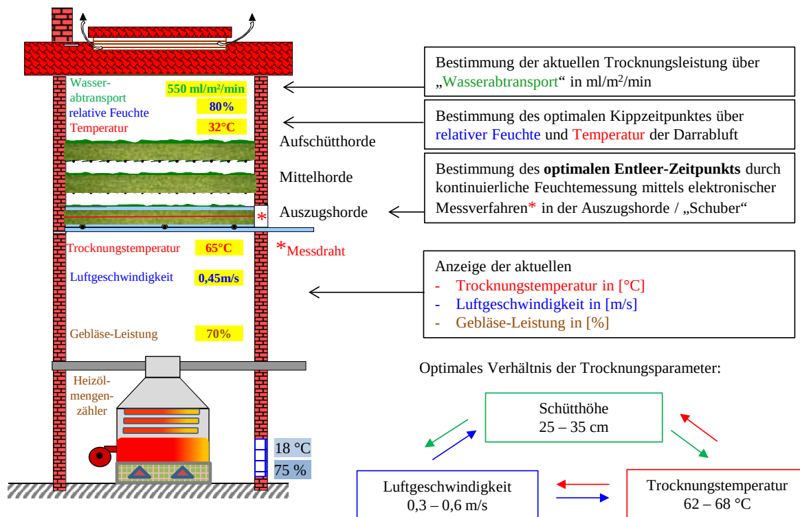
Abb. 50: Wichtige Messwerte in Hopfendarren
