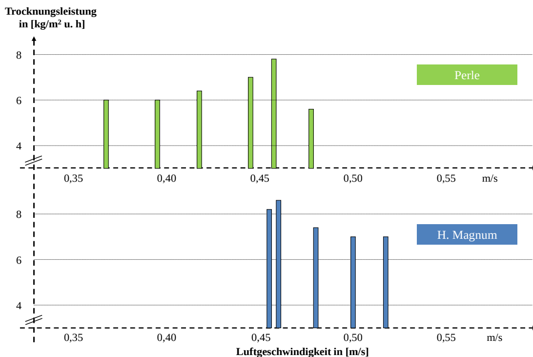
Abb. 66: Trocknungsleistung der Sorten Perle und Hallertauer Magnum in Abhängigkeit von der Luftgeschwindigkeit bei gleichbleibender Schütthöhe
