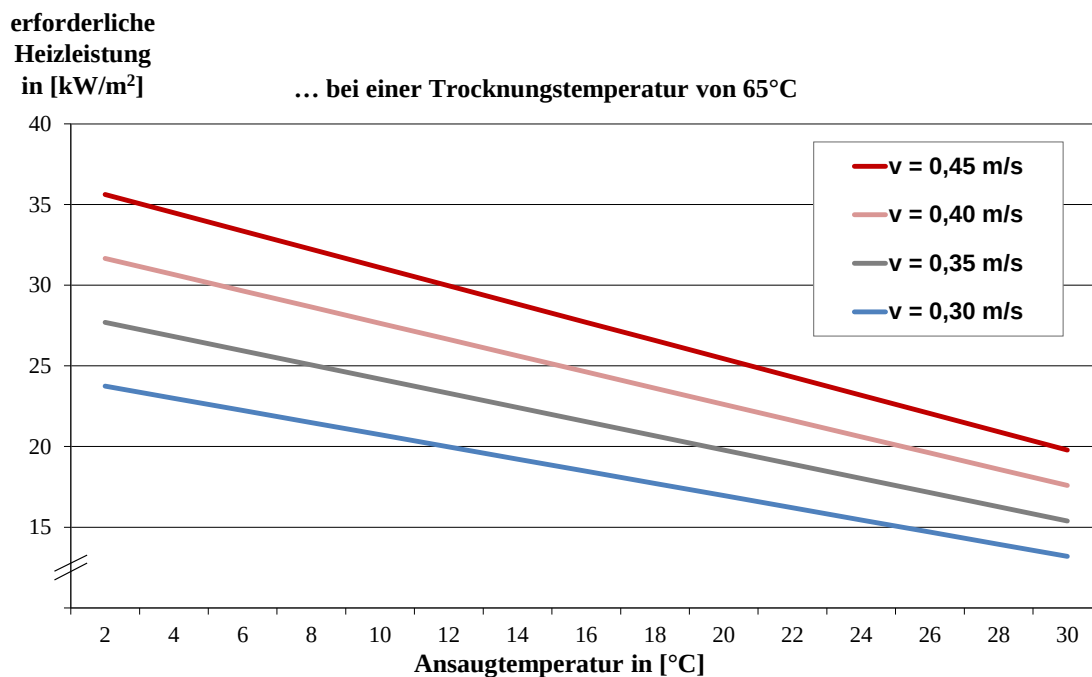
Abb. 5: Erforderliche Heizleistung für eine Trocknungstemperatur von 65^{\circ}\text{C} in Abhängigkeit von Ansaugtemperatur und Luftgeschwindigkeit
