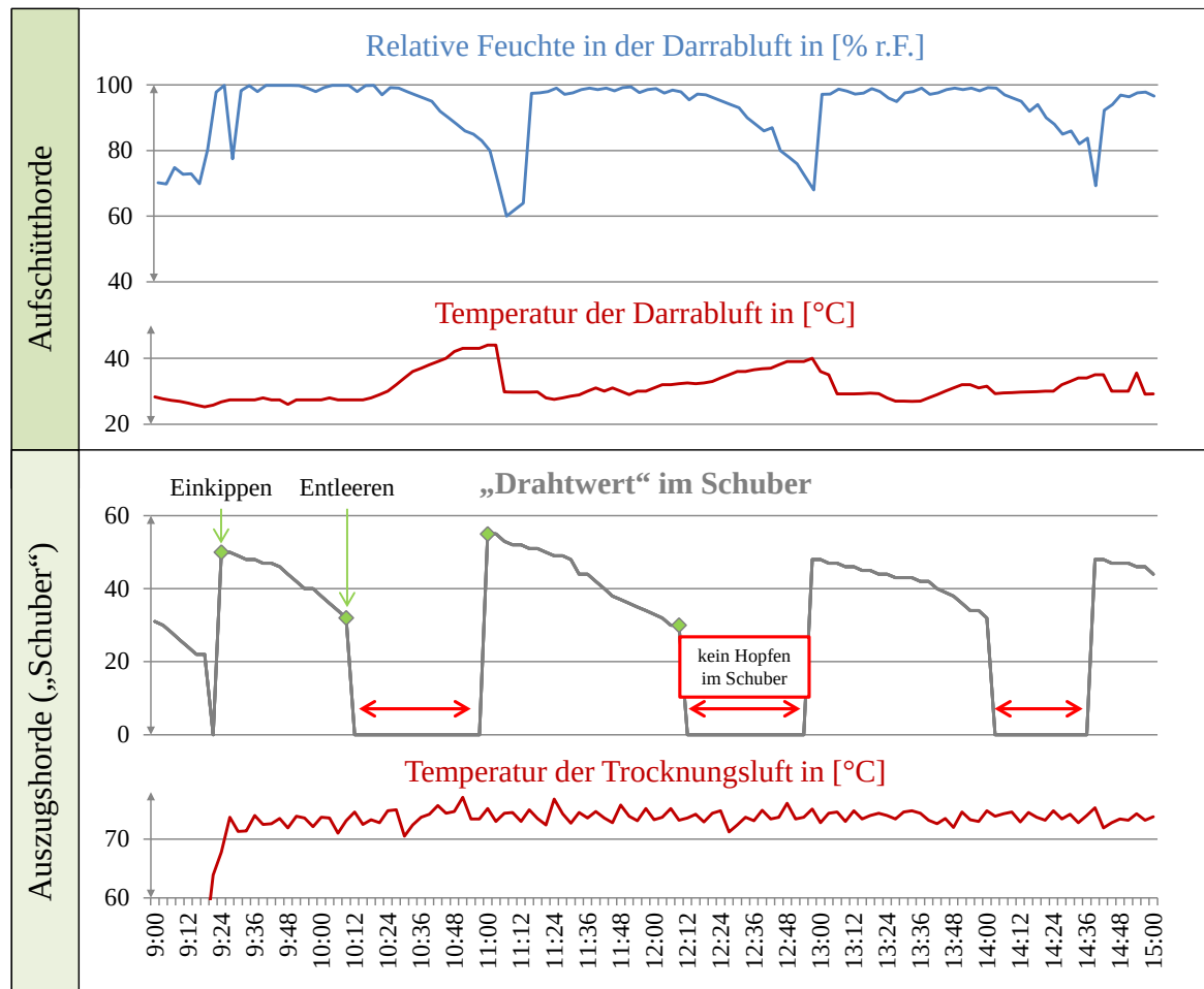
Abb. 59: Graphische Darstellung wichtiger Trocknungsparameter: Beispiel für einen ungleichmäßigen Trocknungsverlauf
