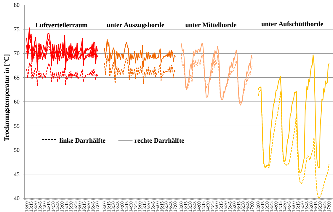
Abb. 11: Trocknungstemperaturen beim Einströmen in die unterschiedlichen Trocknungslagen auf Basis einer ungleichmäßigen Wärme- und Luftverteilung
