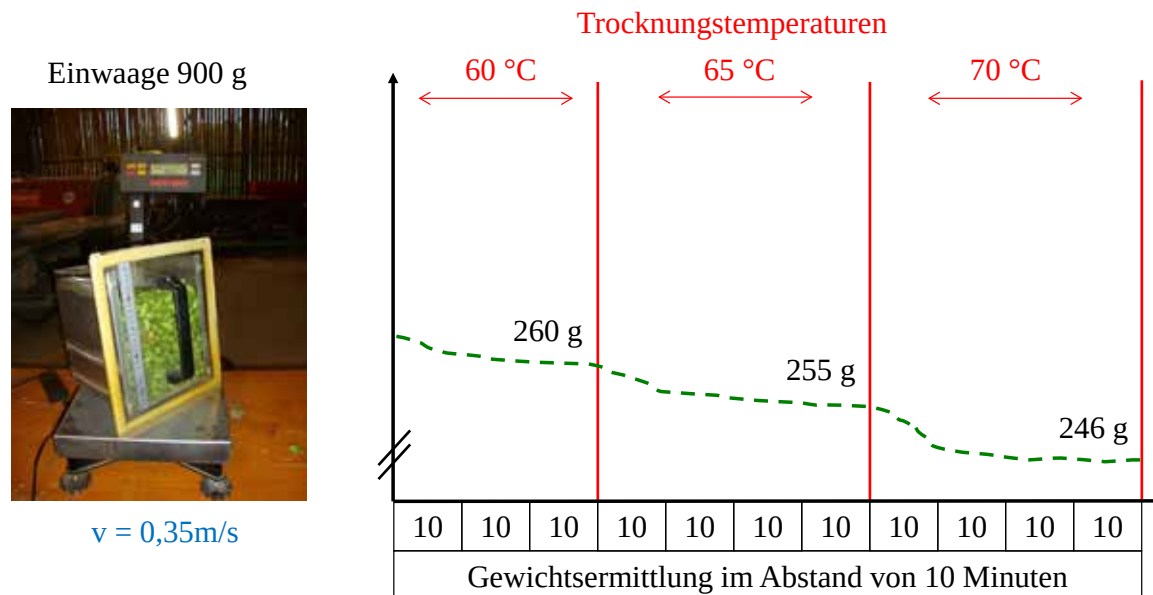
Abb. 22: Kleintrocknungsversuch mit unterschiedlichen Trocknungstemperaturen
