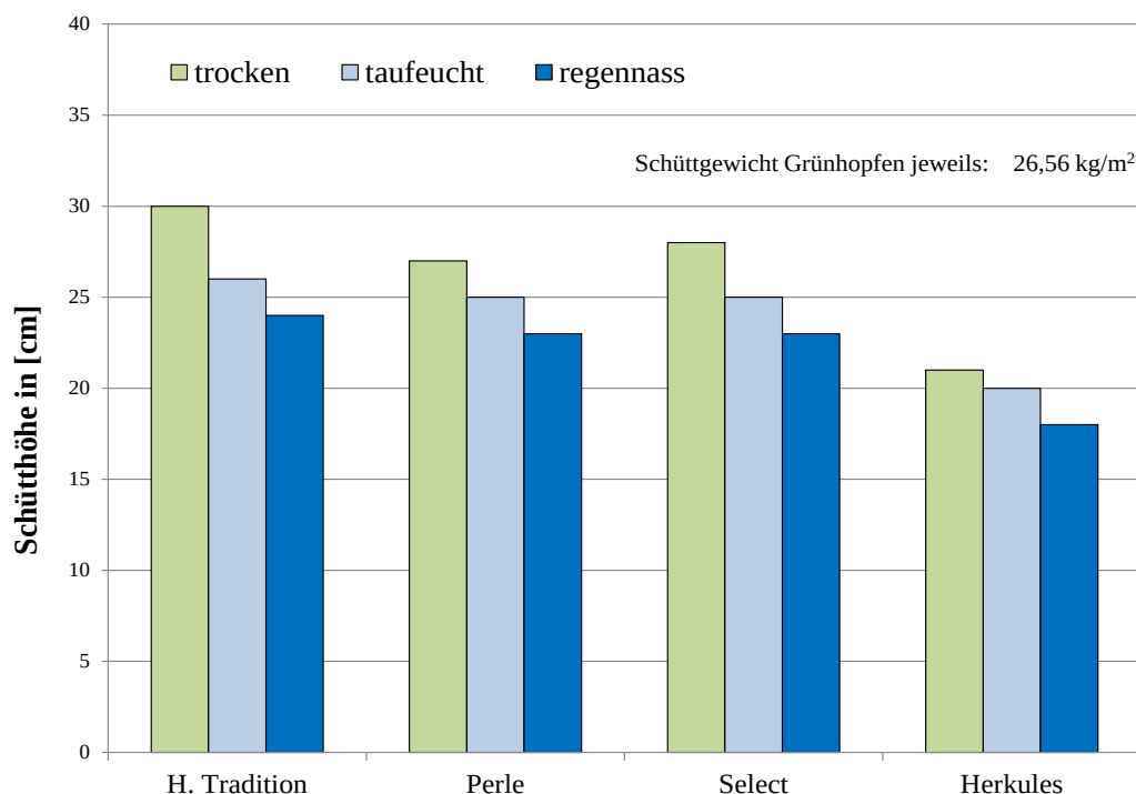
Abb. 47: Schütthöhen bei gleichem Schüttgewicht in Abhängigkeit von Sorte und Feuchtegehalt des Grünhopfens
