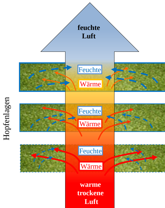
Abb. 16: Schema Wärme- und Wassertransport bei der Konvektionstrocknung
