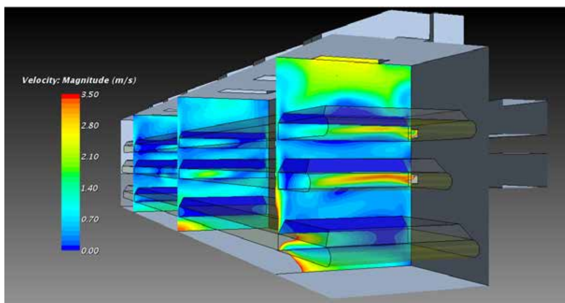
Abb. 12: Strömungssimulation der Trocknungsluft im Bandtrockner tschechischer Bauart (Bild: HTCO GmbH, Freiburg, 2016)
