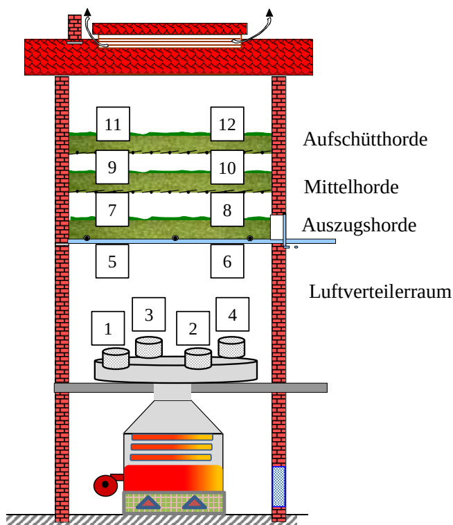
Abb. 9: Positionierung der Data-Logger in Praxisdarren
