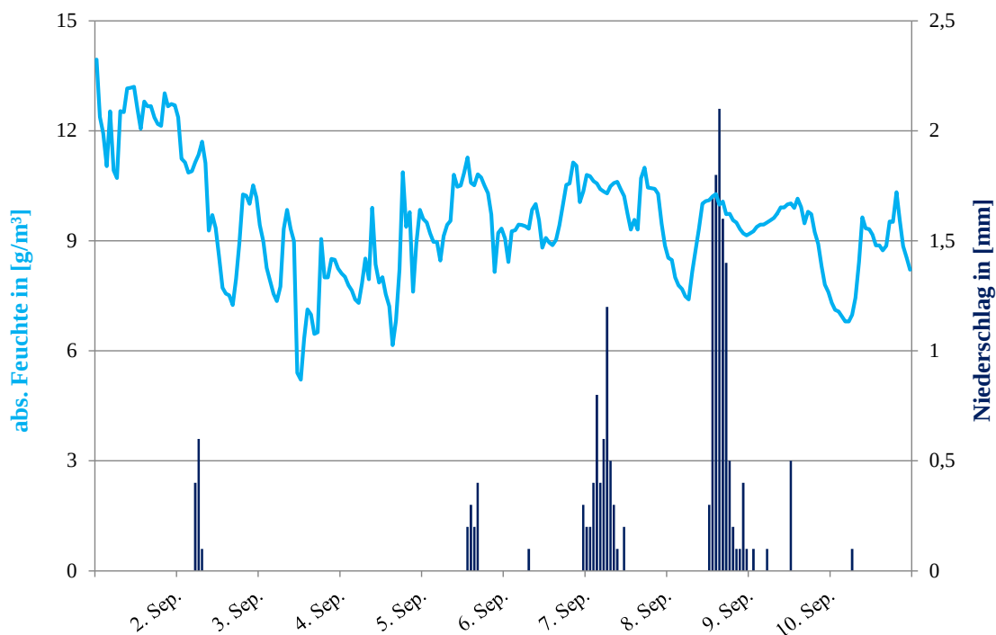
Abb. 42: Veränderung der absoluten Feuchte in der Außenluft während eines Erntezeitraums
