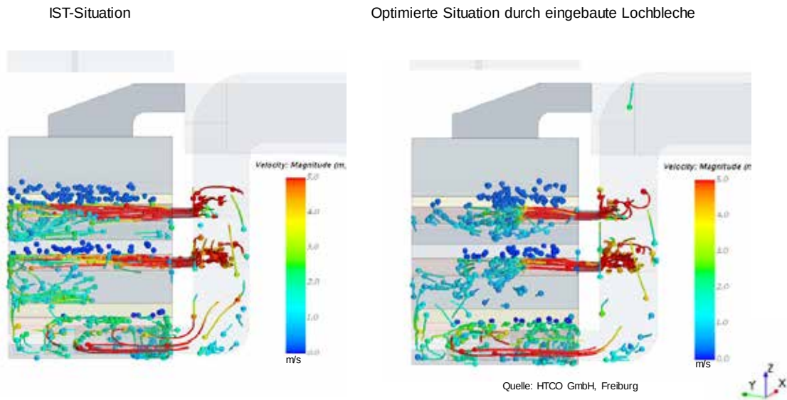
Abb. 13: Darstellung der Strömung der Trocknungsluft im Bandtrockner mittels Strömungslinien in der Querebene (Bild: HTCO GmbH, Freiburg, 2016)
