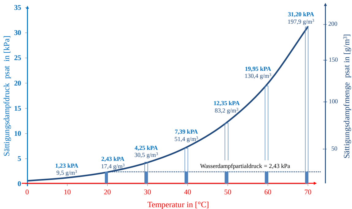
Abb. 19: Zusammenhang von Temperatur, Sättigungsdampfdruck, Wasserdampfpartialdruck und Sättigungsdefizit
