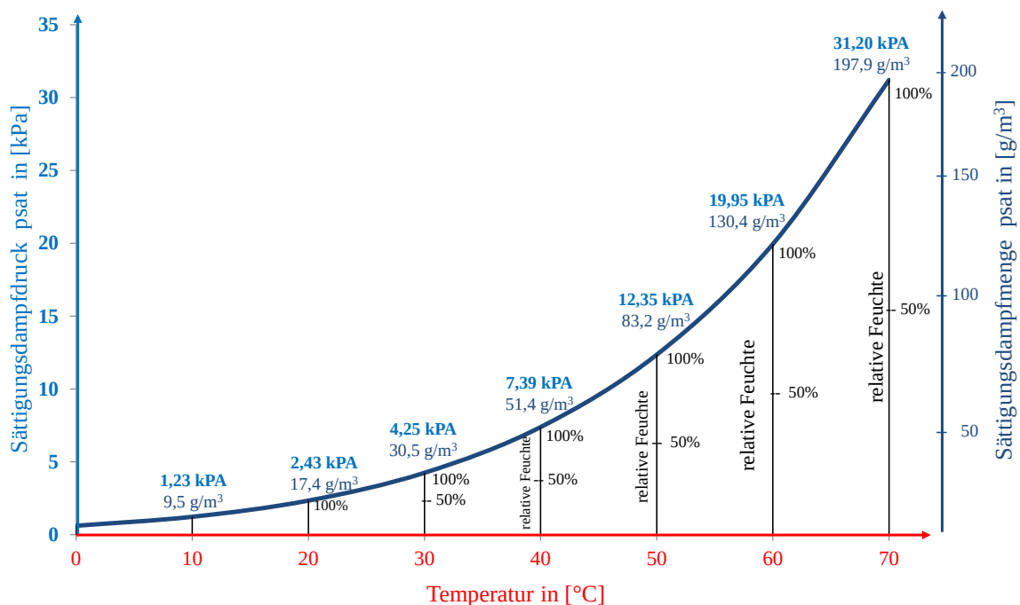
Abb. 18: Zusammenhang von Temperatur, Sättigungsdampfdruck, Sättigungsdampfmenge und relativer Feuchte
