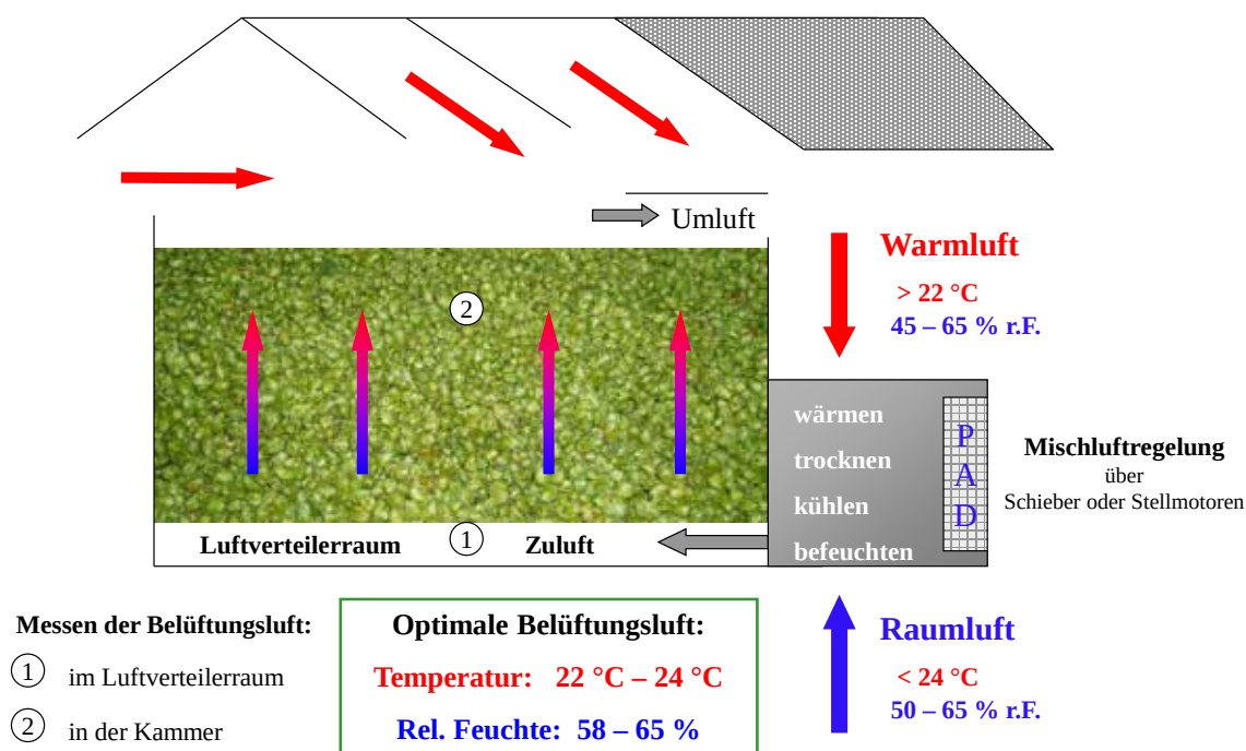
Abb. 77: Schematische Darstellung der Nachbehandlung von Hopfen in Konditionierungskammern
