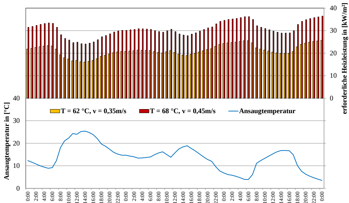
Abb. 6: Veränderung der erforderlichen Heizleistung während eines Erntezeitraums
