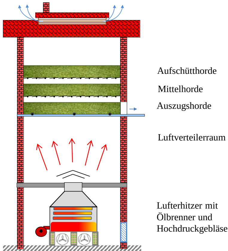
Abb. 1: Schema einer Hopfendarre
