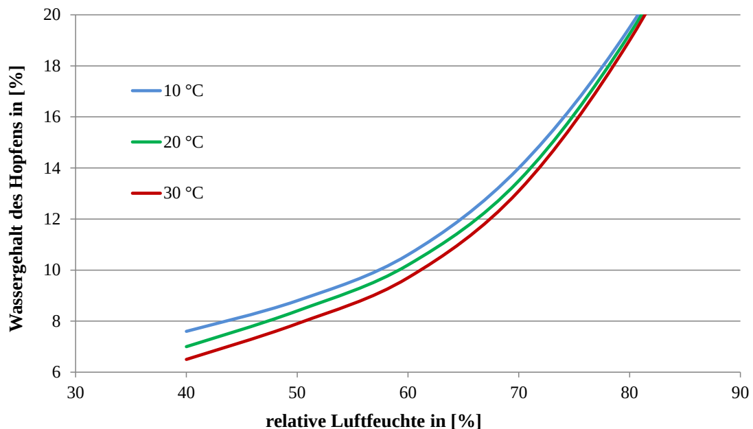
Abb. 21: Sorptionsisothermen von Hopfen
