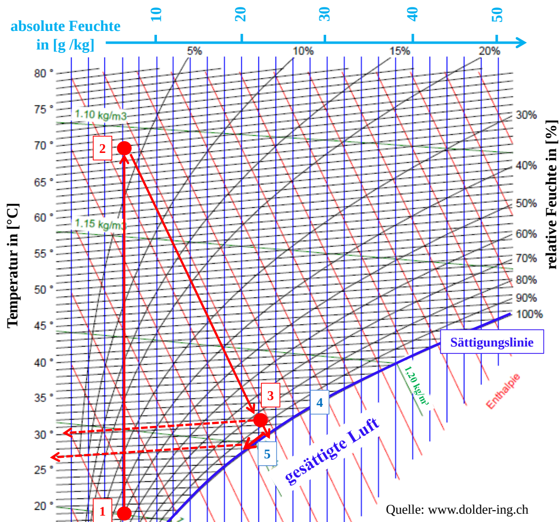
Abb. 17: h_x -Diagramm von Mollier für feuchte Luft
