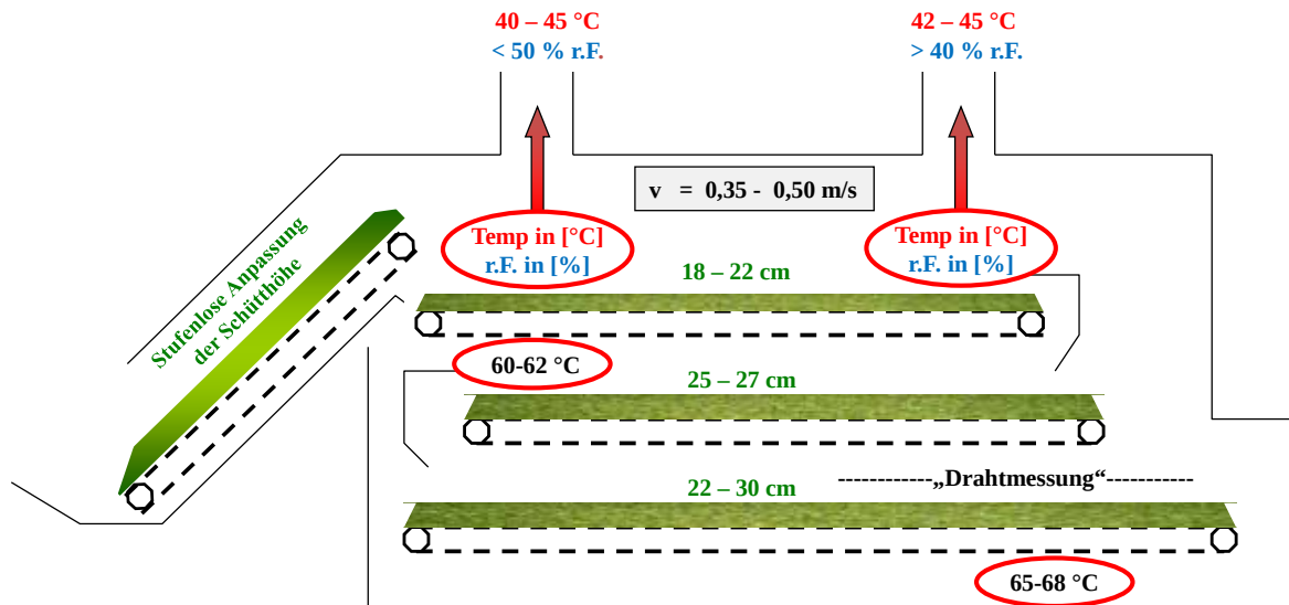
Abb. 61: Messpunkte und mögliche Grundeinstellungen beim Bandtrockner
