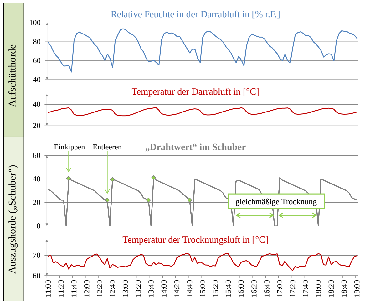
Abb. 58: Graphische Darstellung wichtiger Trocknungsparameter: Beispiel für einen gleichmäßigen Trocknungsverlauf
