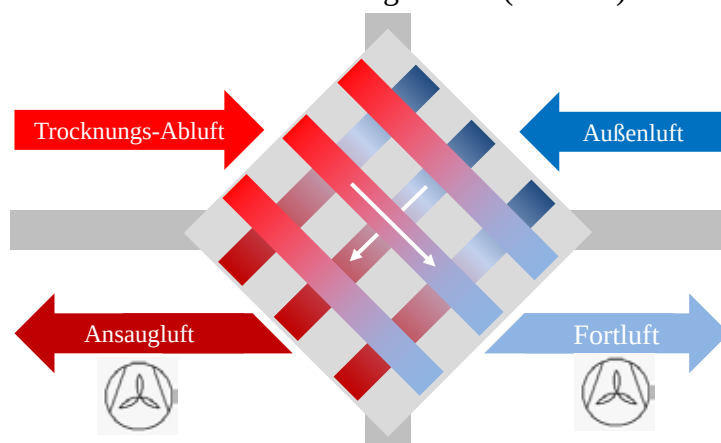
Abb. 75: Prinzip eines Kreuzstrom-Wärmetauschers
