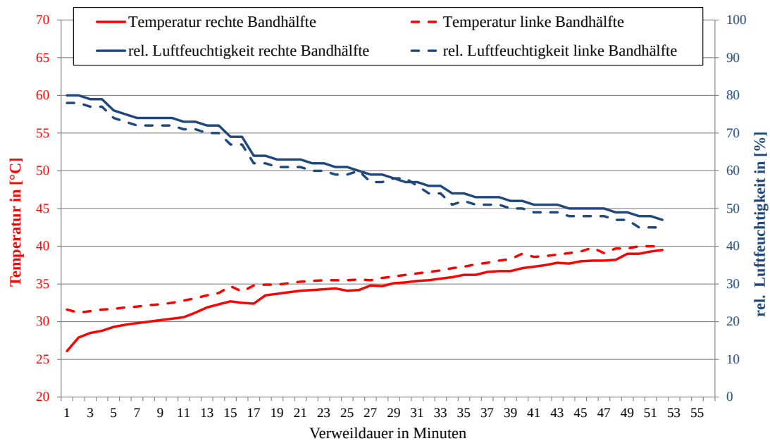
Abb. 15: Veränderung der Temperatur und relativen Feuchte der Abluft aus dem Hopfen im oberen Trocknungsband
