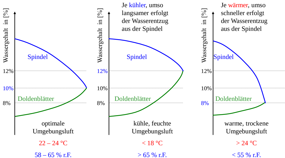
Abb. 79: Feuchteausgleich innerhalb der Dolde nach der Trocknung in Abhängigkeit von der Temperatur
