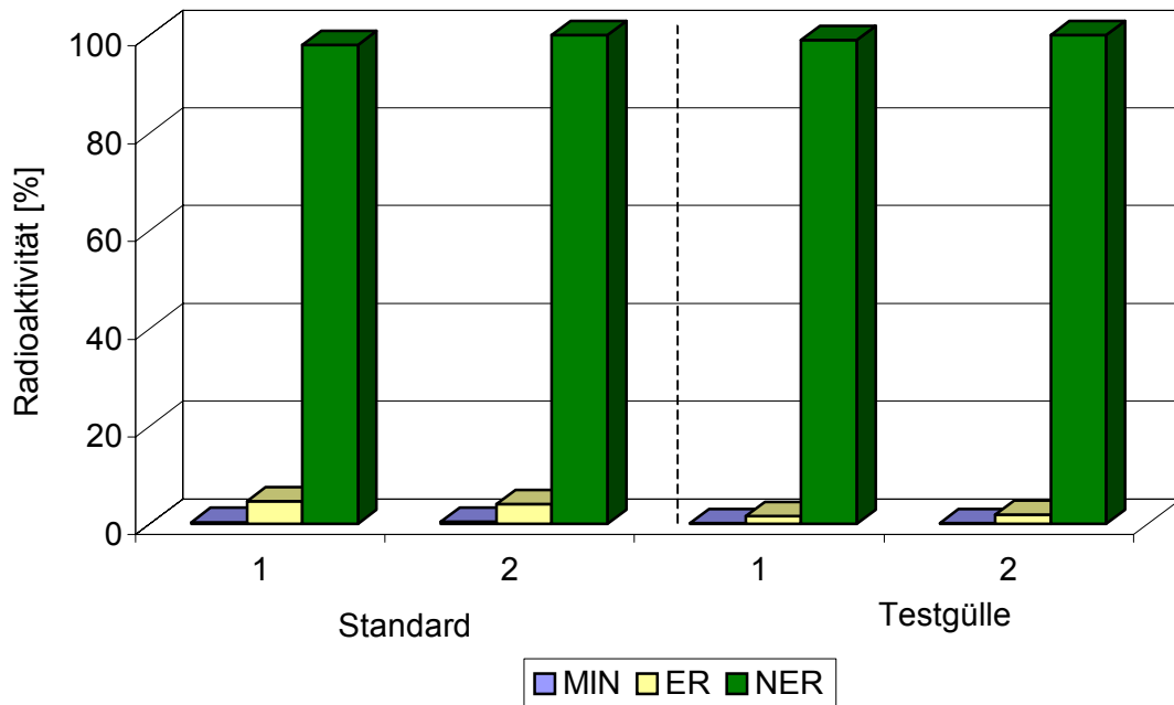
Abb. 4.20: Belebtschlammtest über 28 Tage zur Remobilisierung nicht-extrahierbarer 14 C-Sulfadiazin-Rückstände in schluffigem Tonboden
