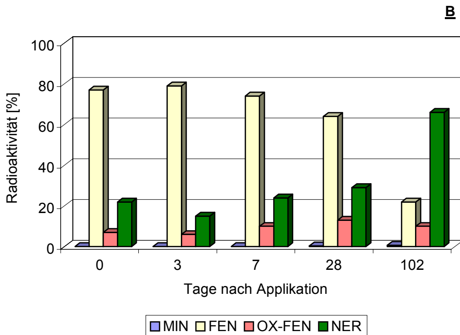
Abb. 4.27: Mikrobieller Abbau von 14 C-Fenbendazol (FEN) A : im schluffigen Ton (AD-A) und B : im schluffigen Sand (NW) nach Testgulle-Applikation unter Beruckichtigung der Metaboliten-Bildung (OX-FEN: Oxfendazol, FEN-SUL: Fenbendazolsulfon)
