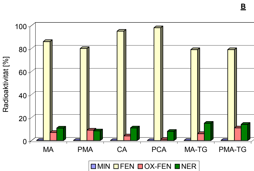
Abb. 4.29: Mikrobieller (MA), chemischer (CA), photoinduziert-mikrobieller (PMA) und photoinduziert-chemischer (PCA) Abbau von 14 C-Fenbendazol (FEN) A : in schluffigem Ton (AD-A) und B : schluffigem Sand (NW) nach Standard- und Testgülle-Applikation (TG)
