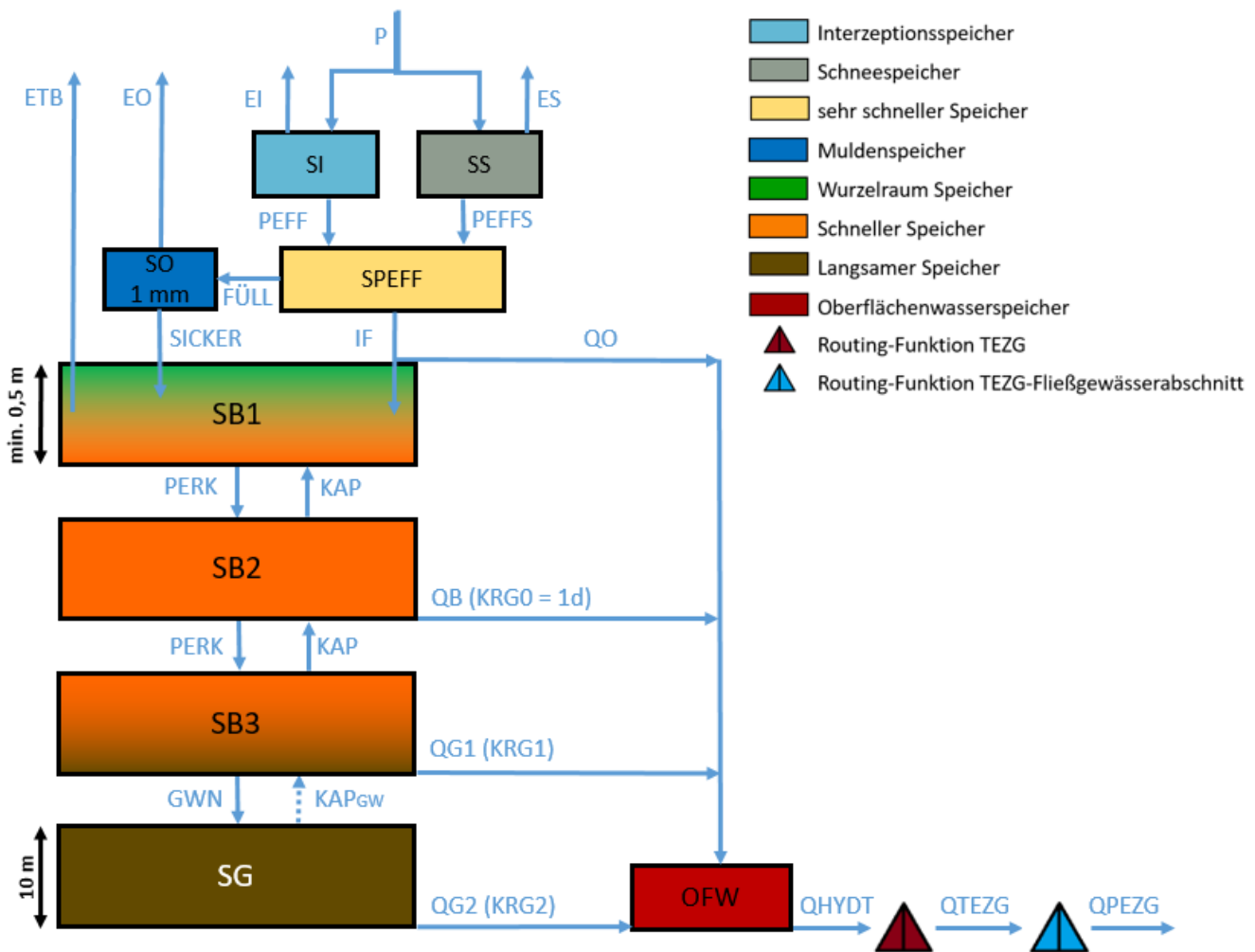
Abbildung 66: Modellstruktur eines Hydrotops für den Anwendungstest in Raven (Darstellung auf Grundlage von (Bouaziz, et al., 2021))
