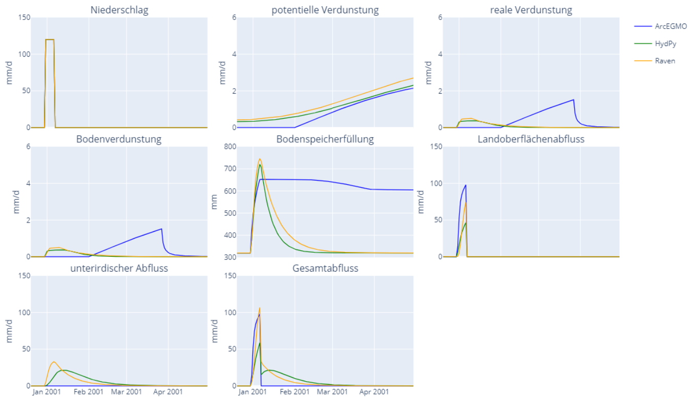
Abbildung 34: Zeitlicher Verlauf ausgewählter Wasserhaushaltsgrößen der drei Basismodelle im Ereigniszeitraum für das Niederschlagsszenario "pblock"
