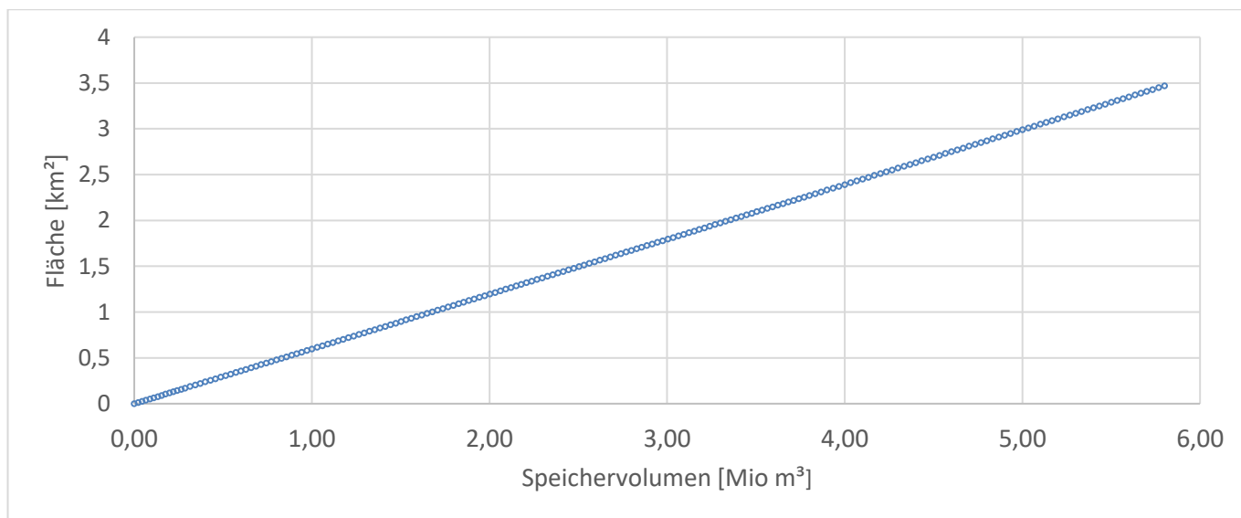
Abbildung 61: Lineare Zunahme der Wasserfläche mit dem Speichervolumen des Speichers Lohsa I
