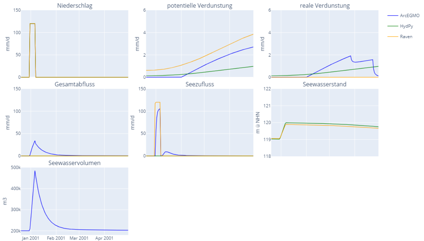
Abbildung 50: Reaktion des ungesteuerten Reservoirs in ArcEGMO, HydPy und Raven auf das Niederschlagsszenario "pblock" unter Berücksichtigung der Seeverdunstung innerhalb des kF-Tests
