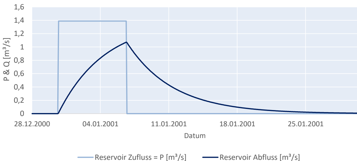
Abbildung 51: Reaktion des ungesteuerten Reservoirs in Raven auf das Niederschlagsszenario "pblock" ohne Berücksichtigung der Seeverdunstung innerhalb des kF-Tests
