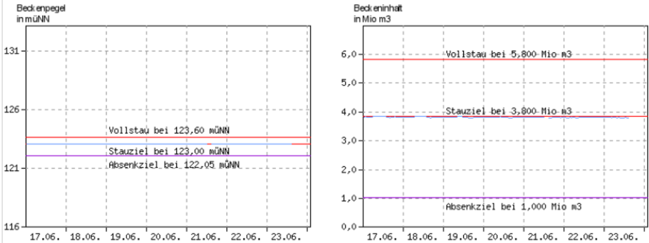
Abbildung 58: Stauziele des Speicherbeckens Lohsa I
