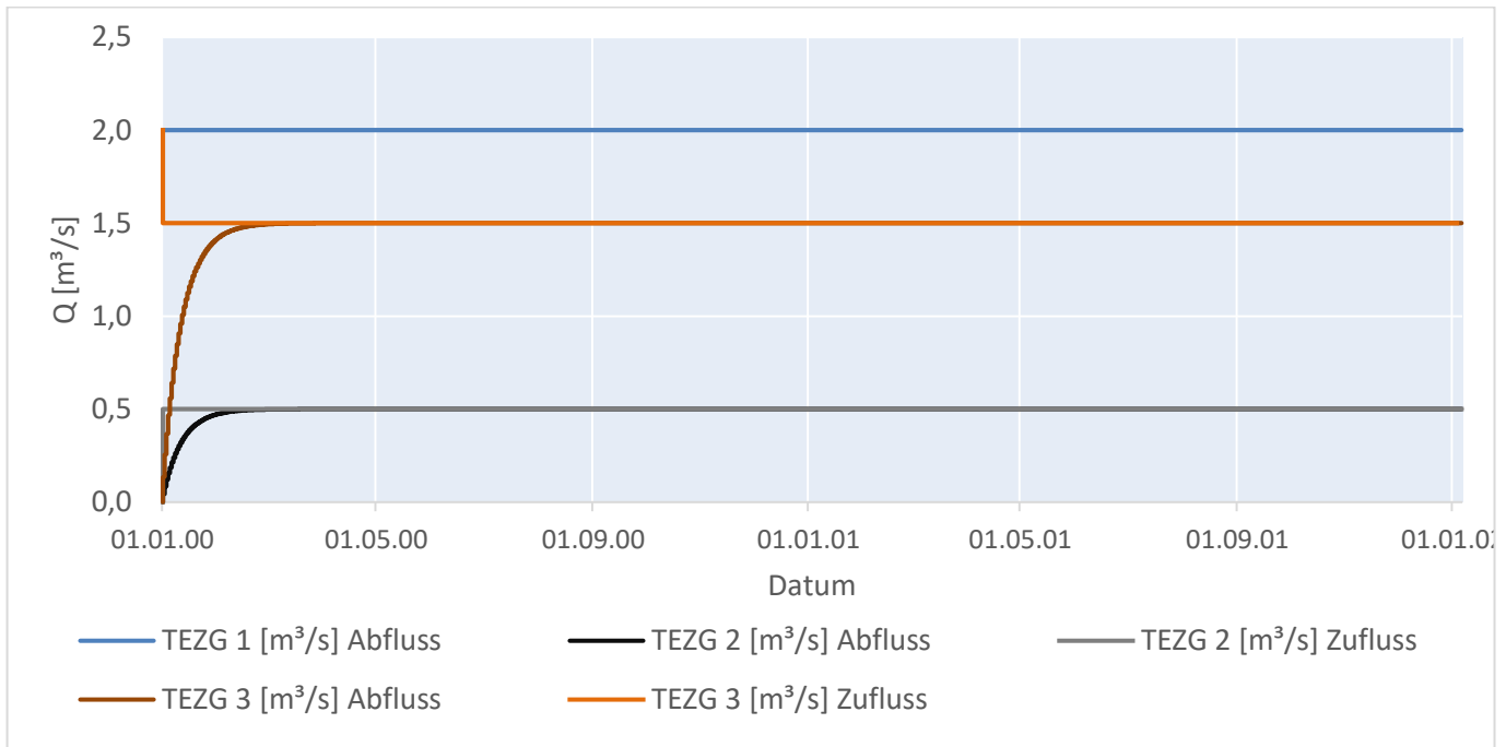
Abbildung 56: Ergebnisse des bS-Tests in Raven mit Aufteilung des Abflusses aus TEZG 1 auf TEZG 2 und TEZG 3 für FlowDiverison und FlowDiverison mit Lookup-Tabelle (ohne Seeverdunstung in TEZG 2 und TEZG 3)
