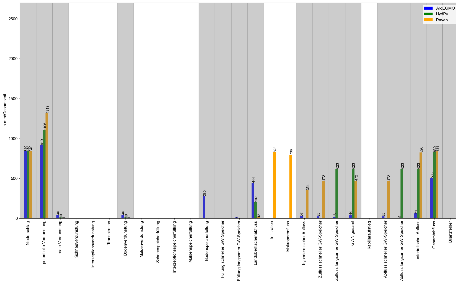
Abbildung 43: Vergleich der Wasserhaushaltsbilanzen in mm/Gesamtzeitraum (ca. zwei Jahre) für die cF-Modelle (Landnutzung unbewachsener Boden, Bodenart Ls3) und das Niederschlagsszenario "pblock" (alle hier relevanten und in jedem Modell als Ausgabewerte verfügbaren Wasserhaushaltsgrößen sind grau hervorgehoben)
