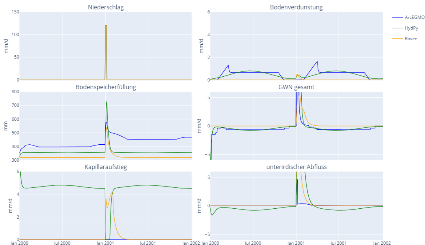
Abbildung 46: Zeitlicher Verlauf ausgewählter Wasserhaushaltsgrößen der drei cF-Modelle im Gesamtzeitraum für das Niederschlagszenario "pblock" (Landnutzung unbewachsener Boden, Bodenart Ls3), im Nichtereigniszeitraum entspricht "GWN gesamt" dem Kapillaraufstieg in ArcEGMO
